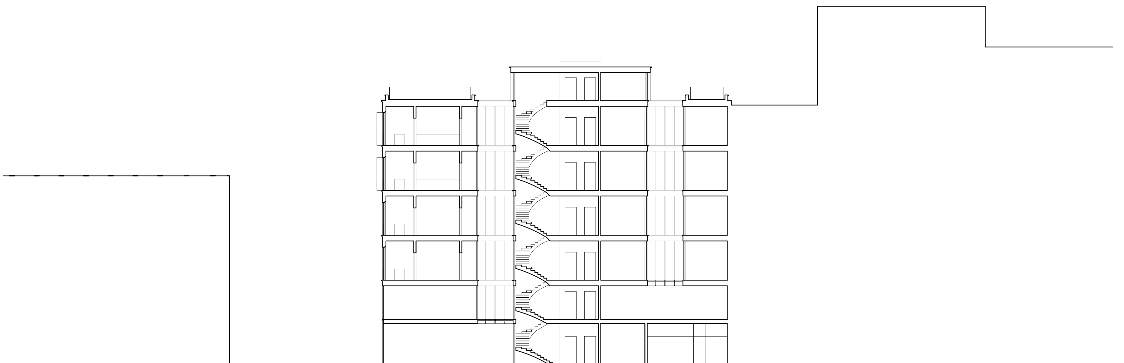
SCHNITT BB | 1:200
