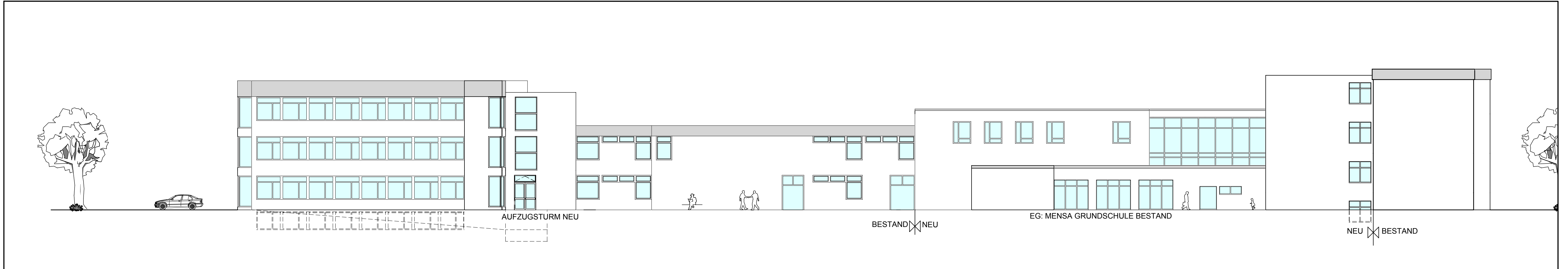
ANSICHT NORD M 1 : 200
