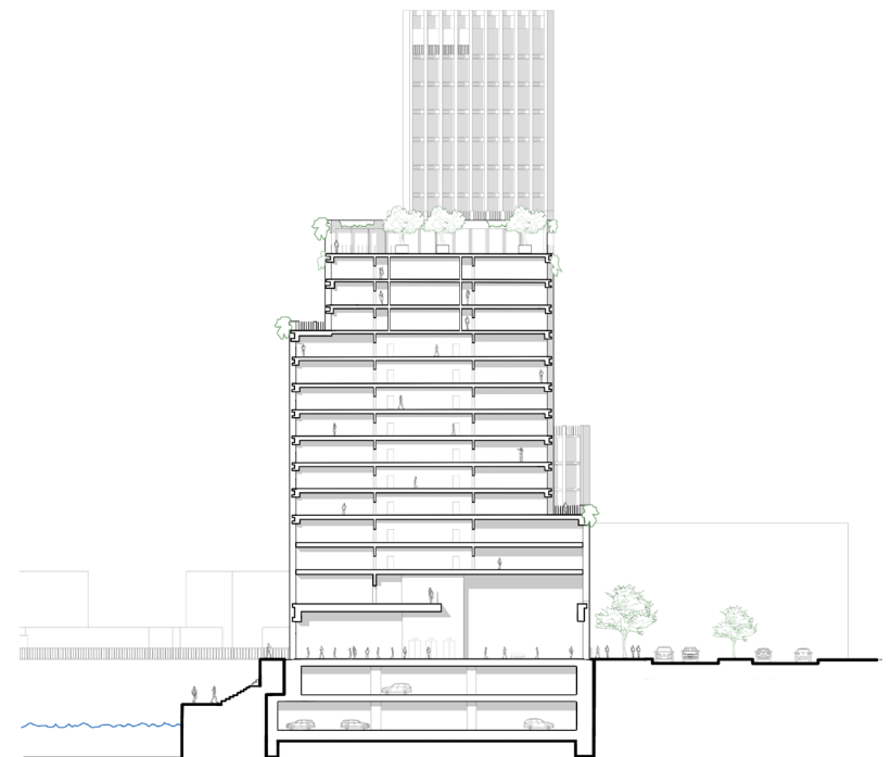
schnitt m 1:500
