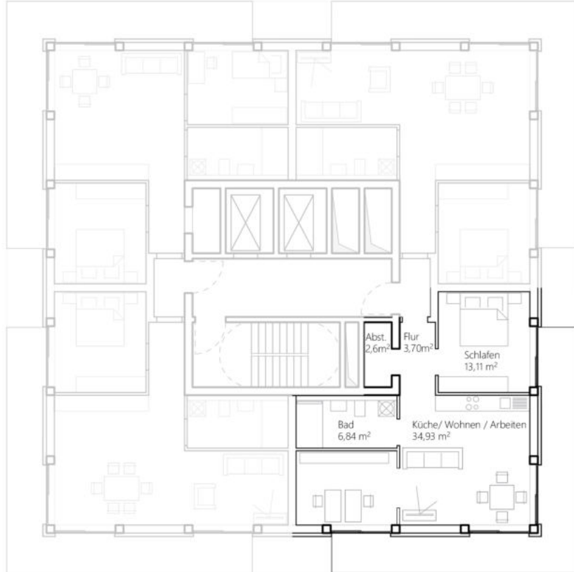
GRUNDRISS VARIANTE 1 | M 1.200 ⌚ 4x 2-ZIMMER-WHG (GROß)
