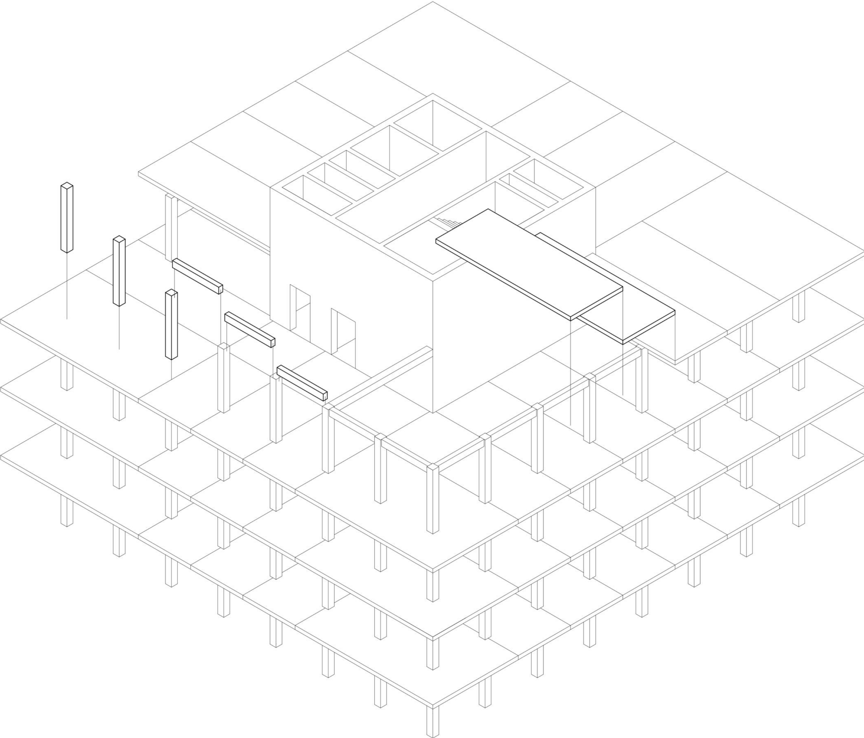
SCHEMATISCHER AUFBAU DER HOCHHÄUSER
