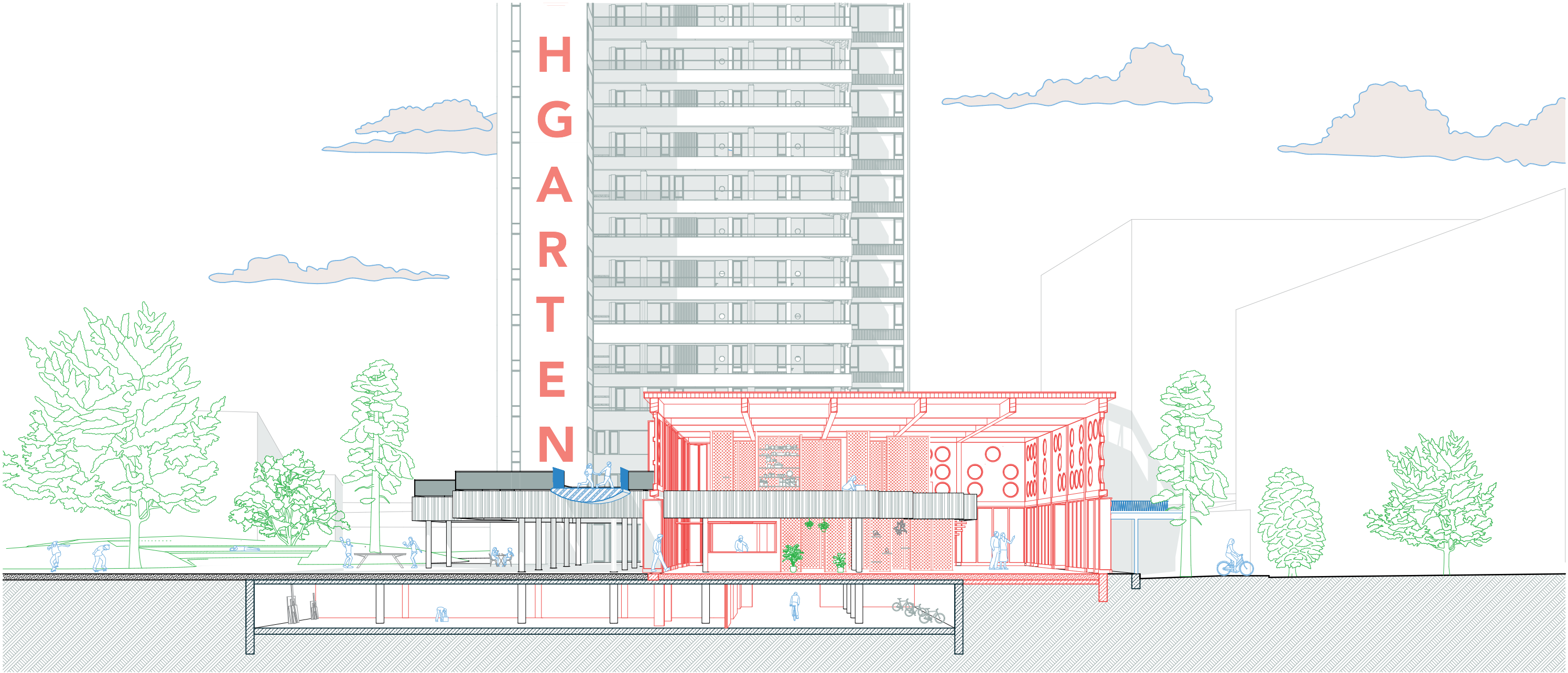
3 D Schnitt M 1:200
