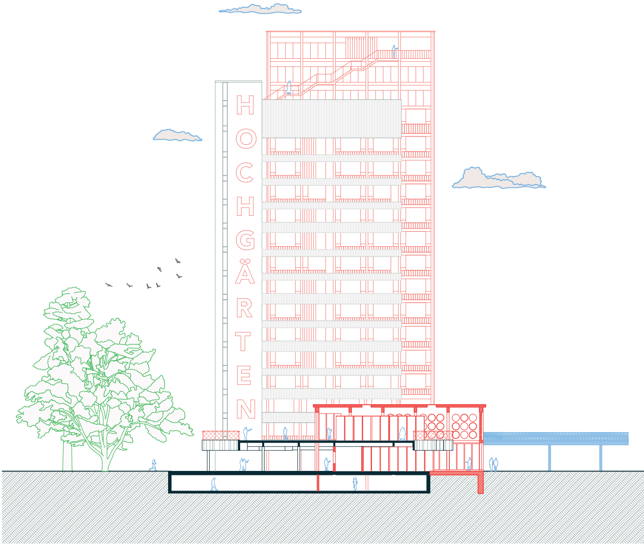
Schnitt B-B M 1:500
