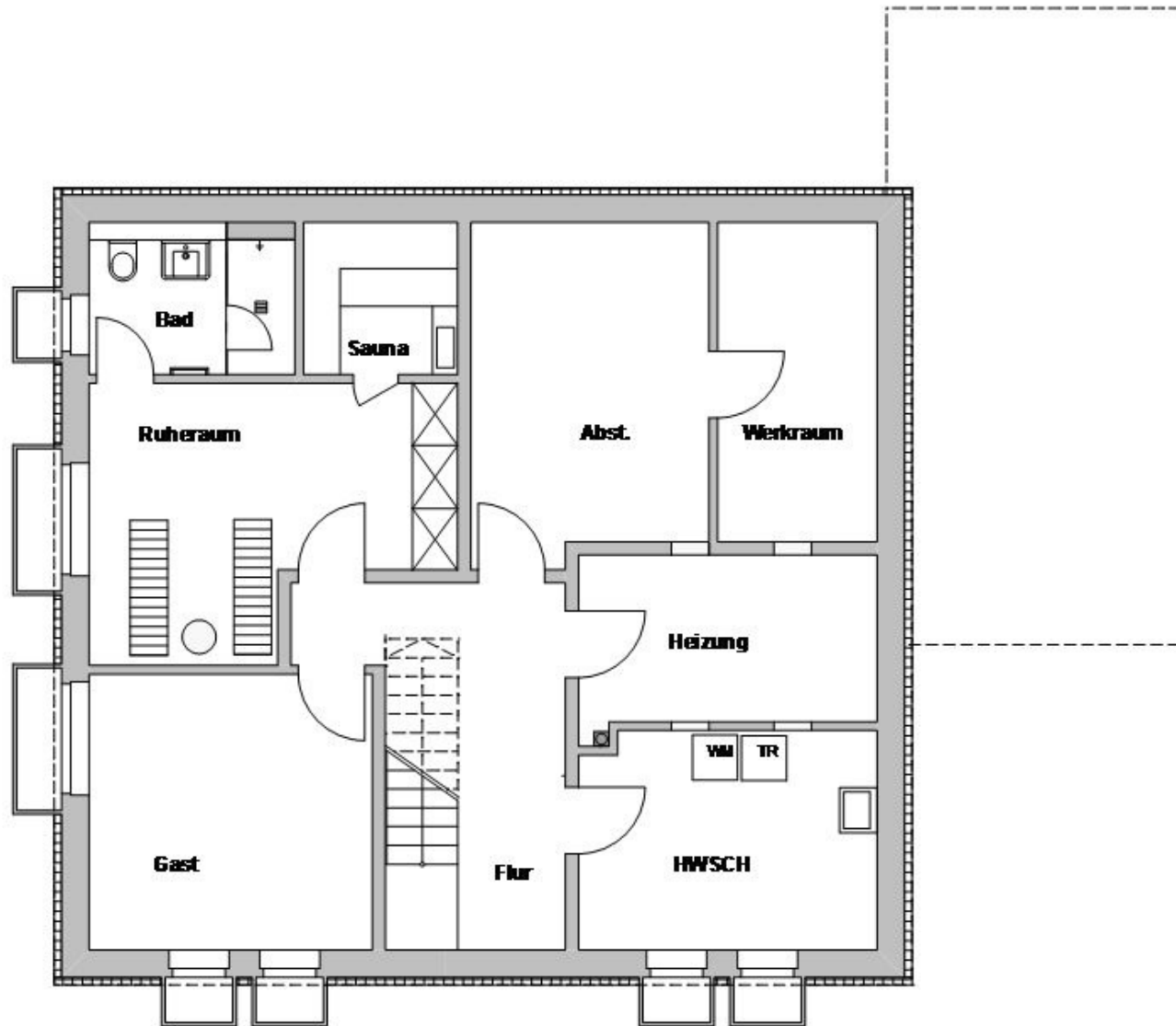
Kellergeschoss
