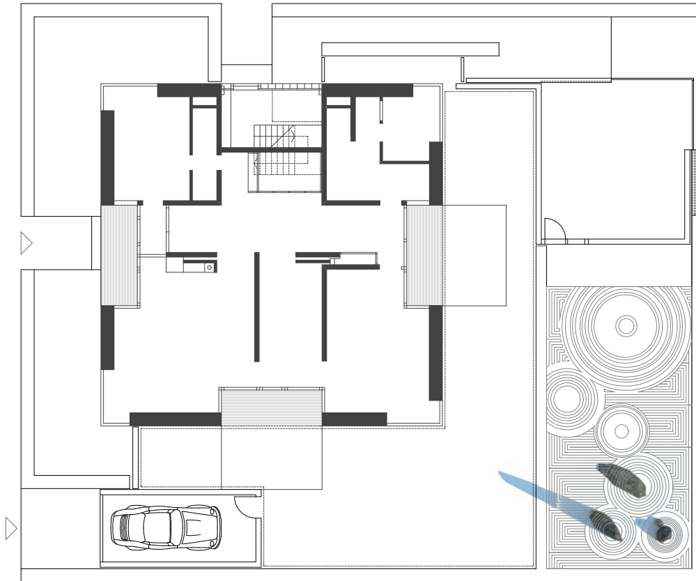
Grundriss EG M 1: 200
