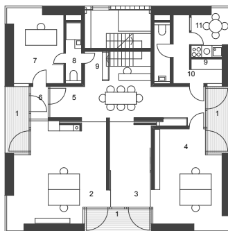
EG ( Variante A : Büro )
