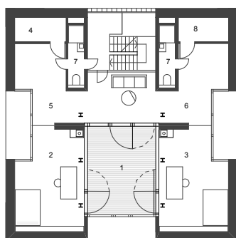
2OG ( Variante A : Kinderzimmer )
