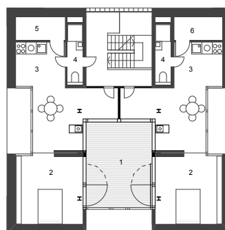
Grundriss 2 OG M 1: 200
