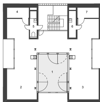
2OG ( Variante D : Atrium )
