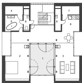
2OG ( Variante C : Wohnung )
