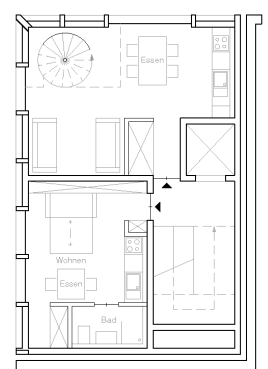
IV. Obergeschoss
