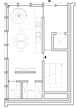
Erdgeschoss
