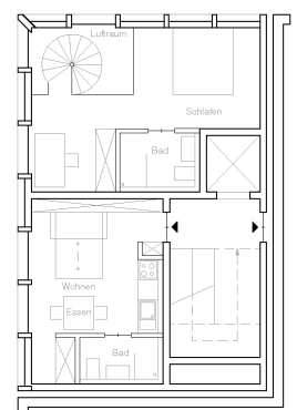
III. Obergeschoss
