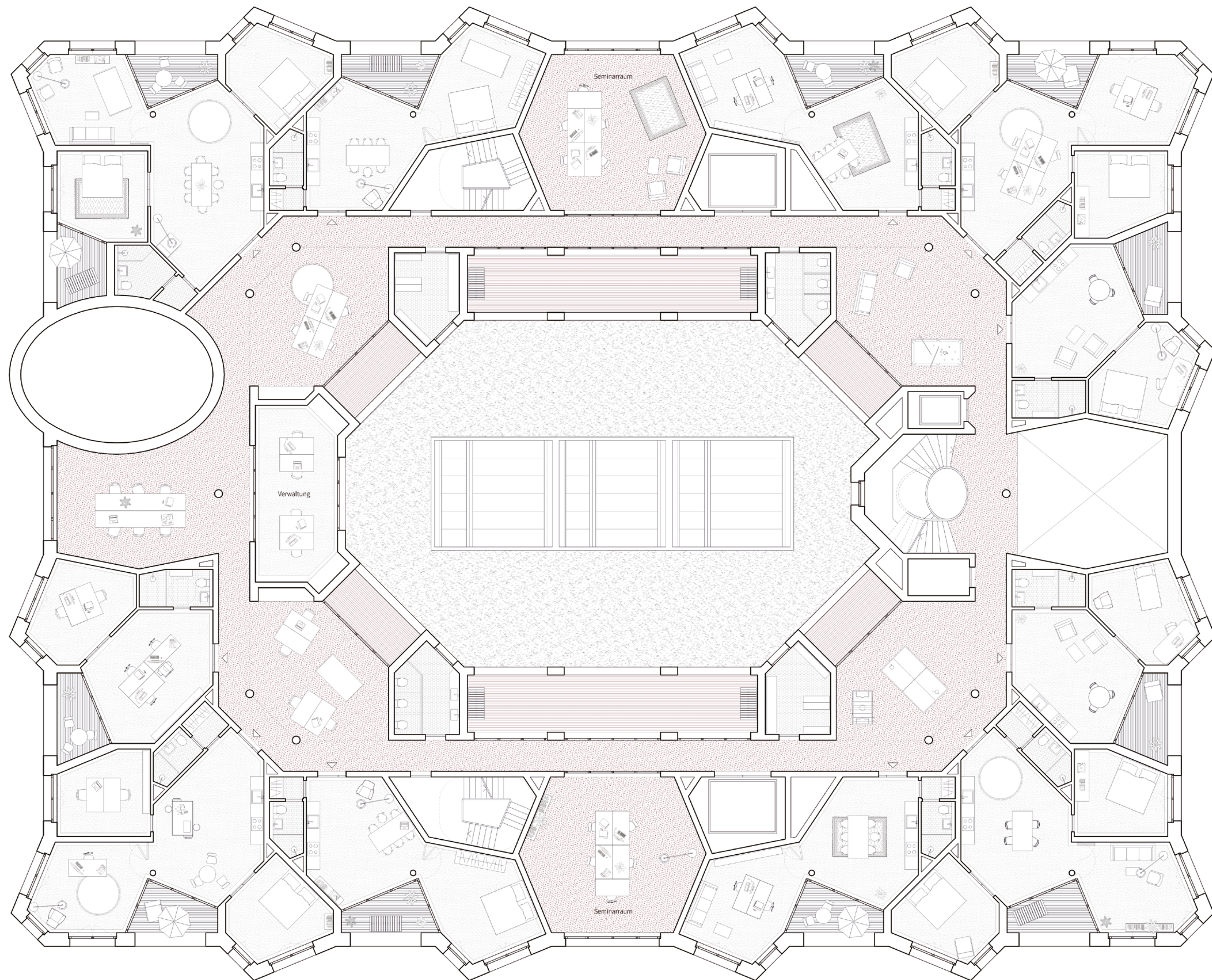
Grundriss 1. Obergeschoss M 1:100
