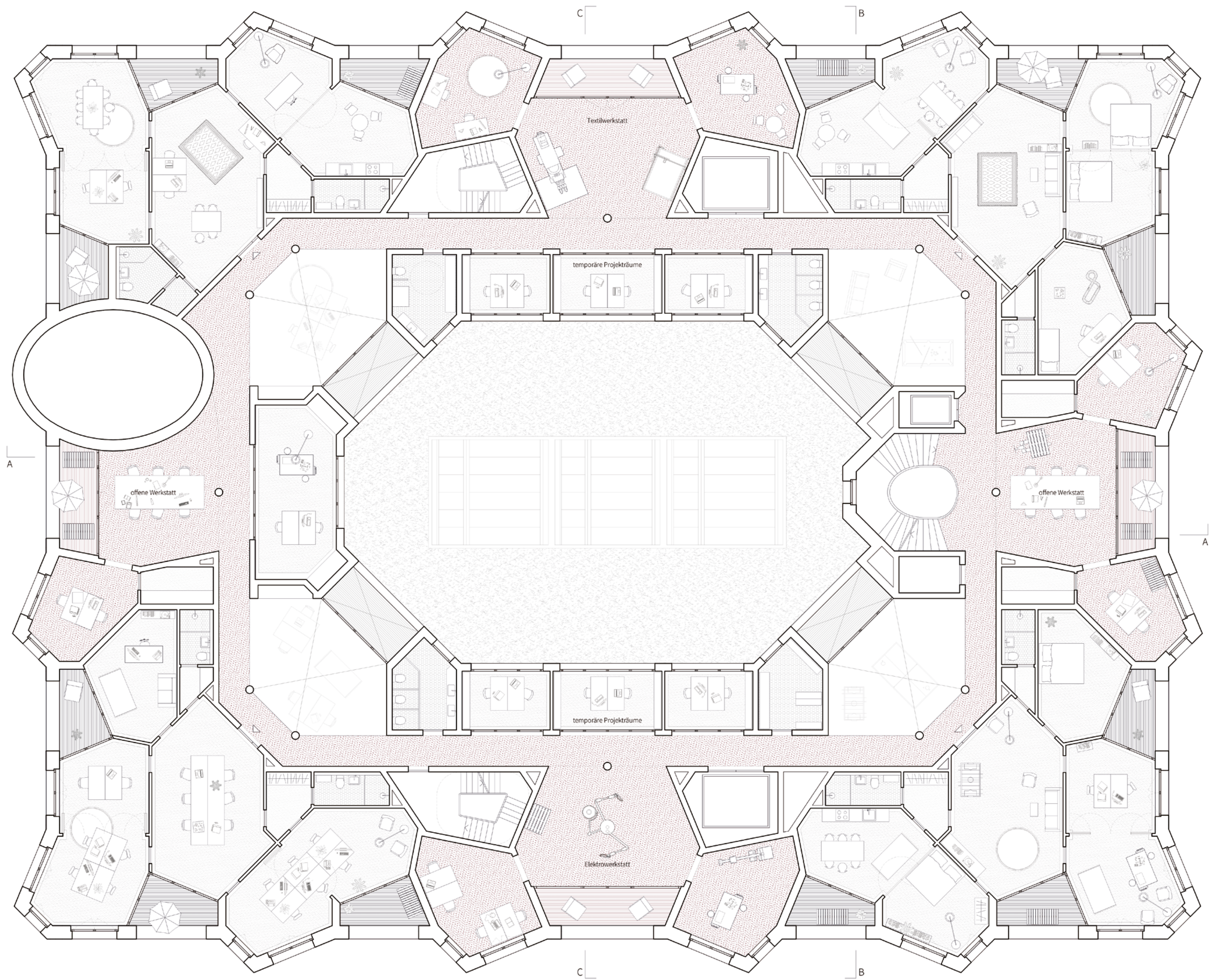
Grundriss 2. Obergeschoss M 1:100
