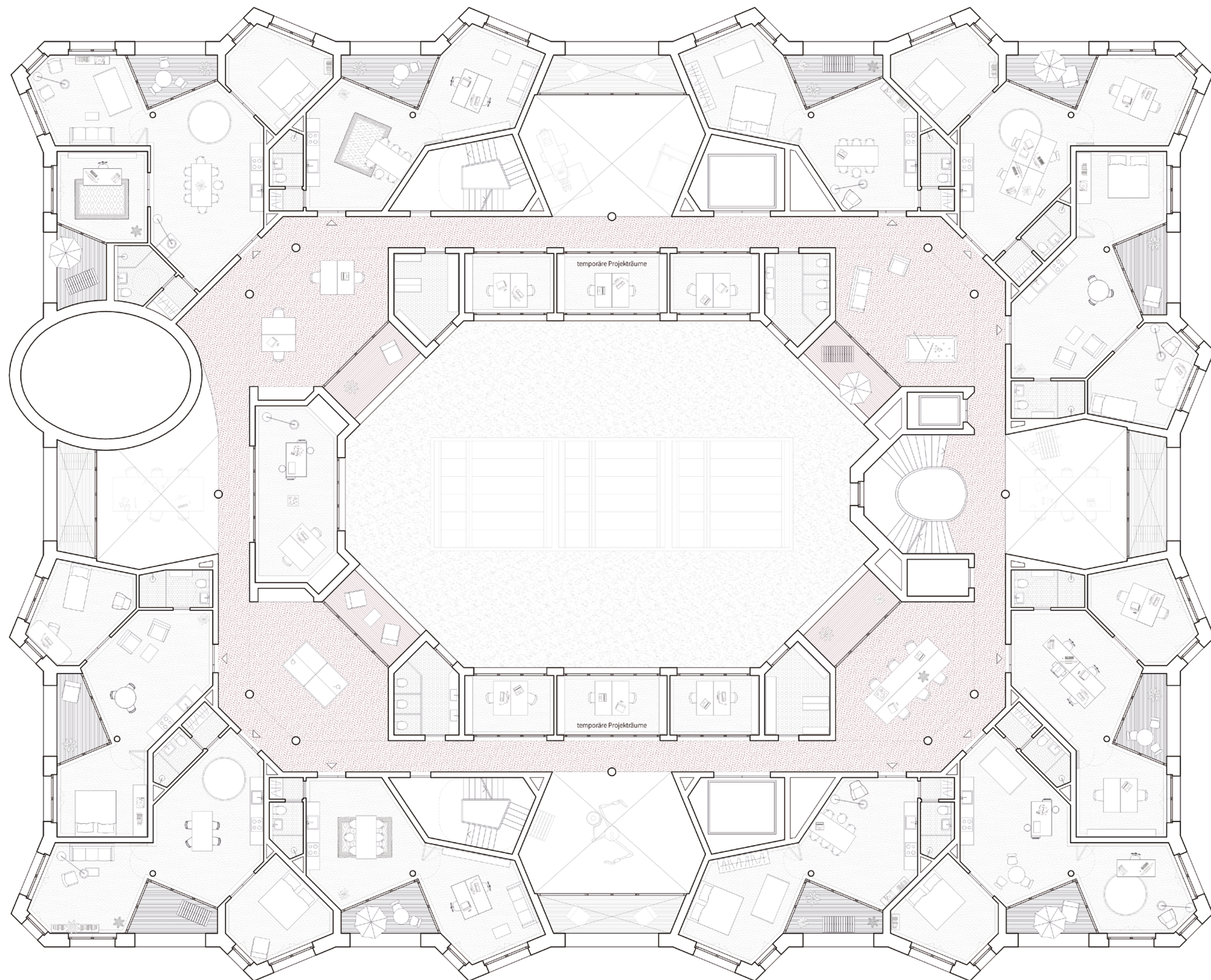
Grundriss 3. Obergeschoss M 1:100
