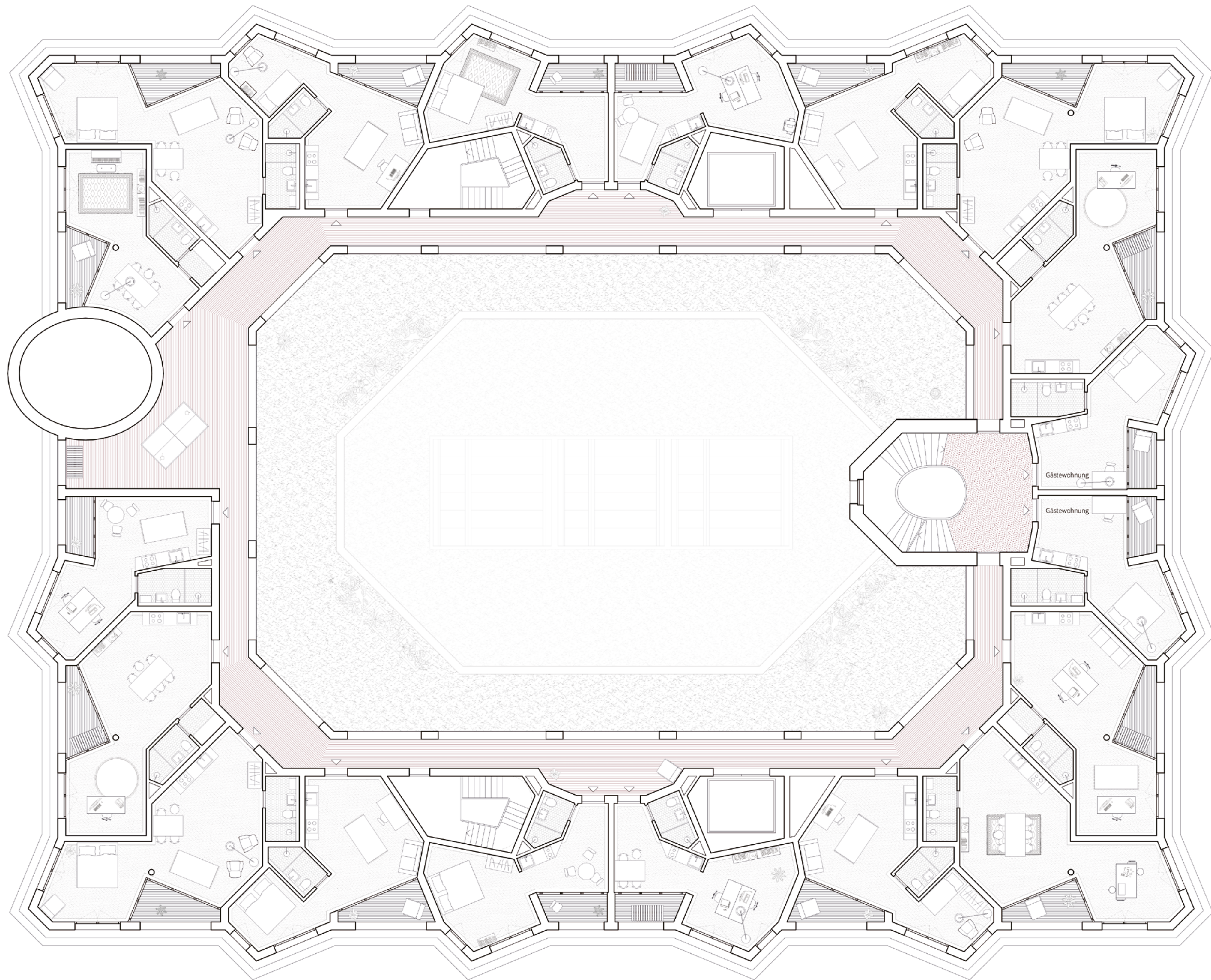
Grundriss 7. Obergeschoss M 1:100
