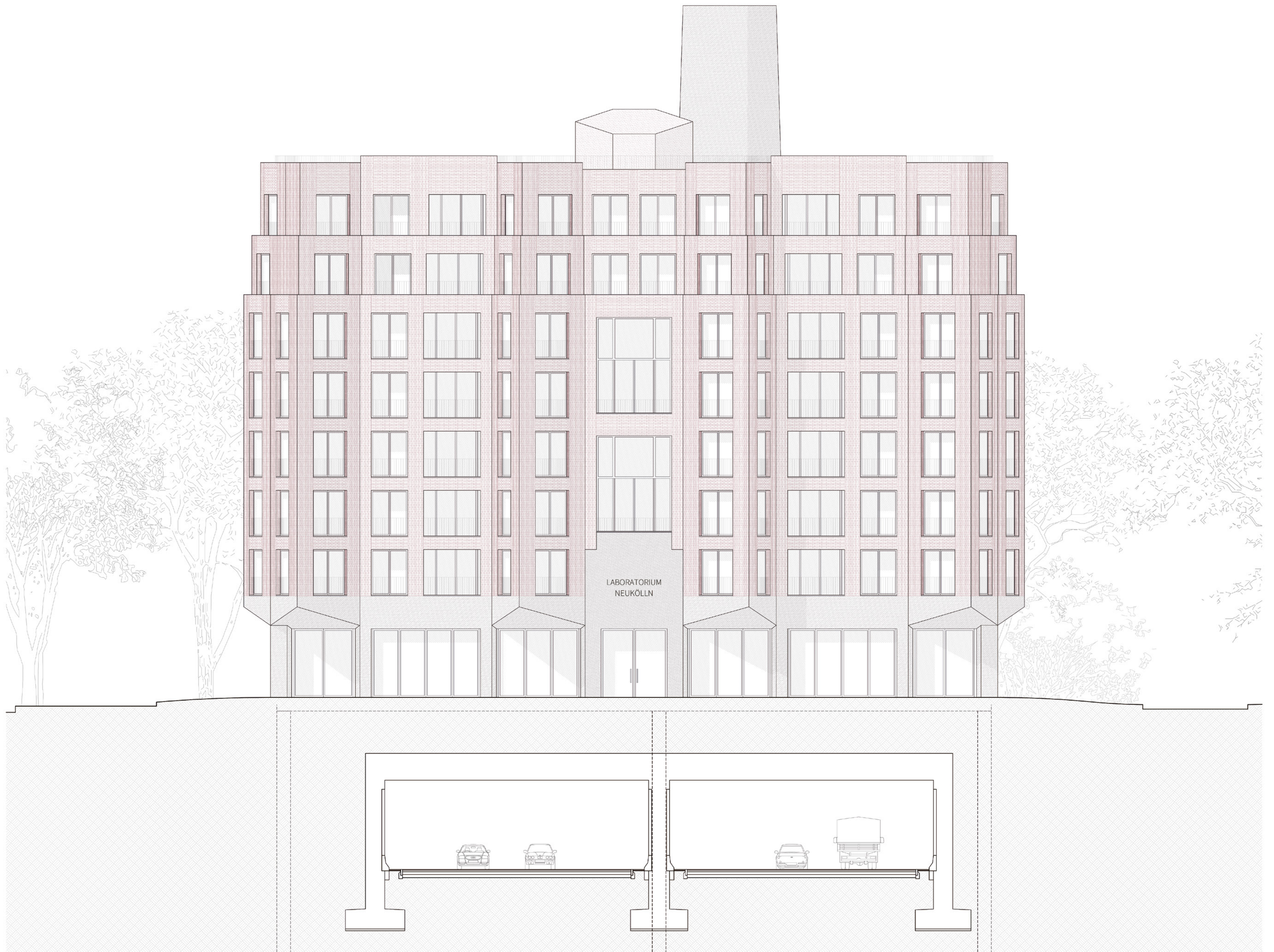
Ostansicht M 1:100
