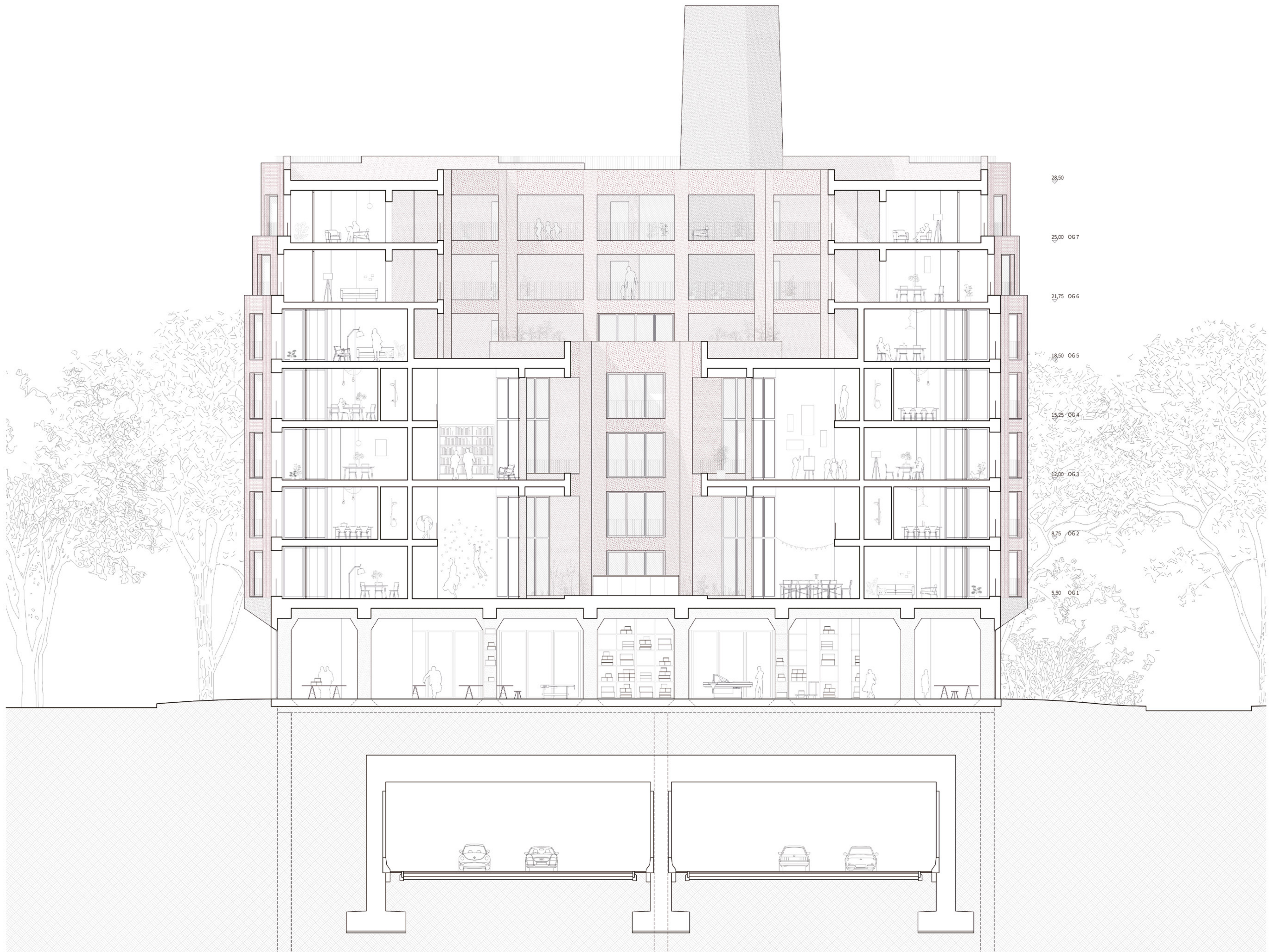
Schnitt B M 1:100
