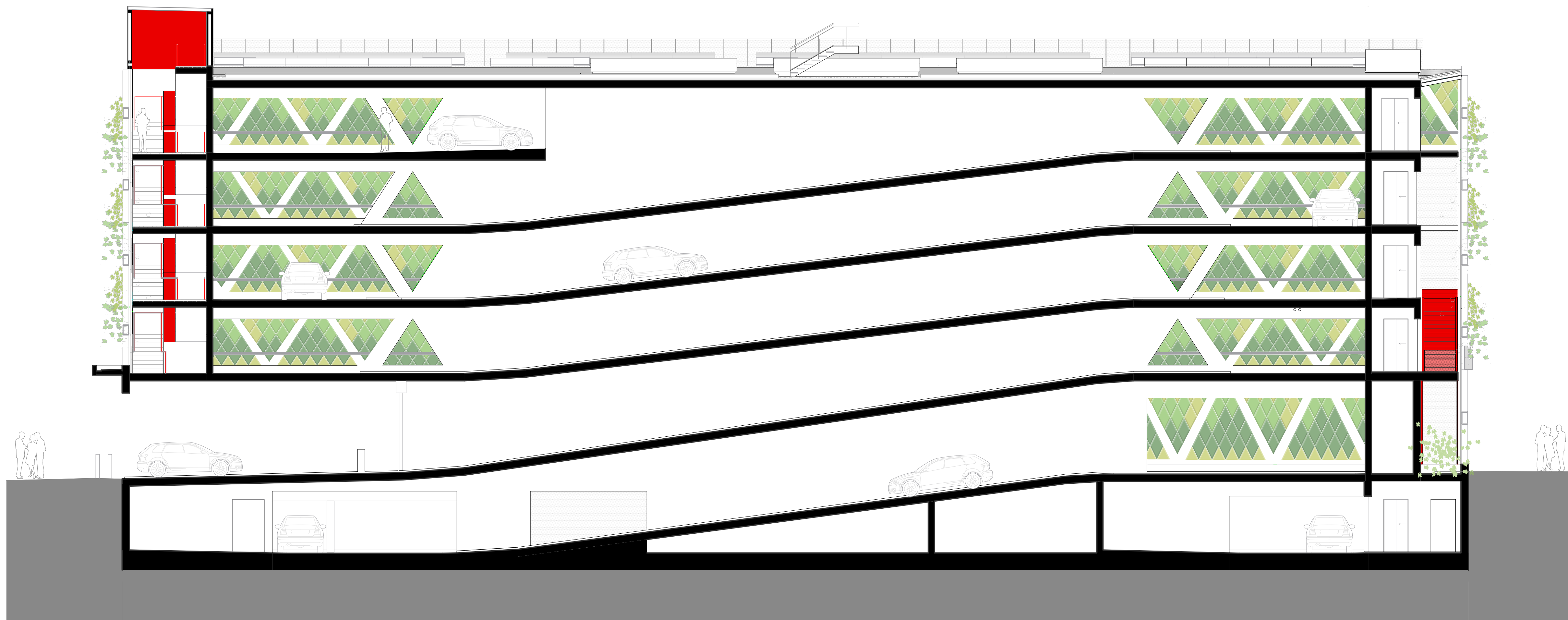
Schnitt A-A 1:100
