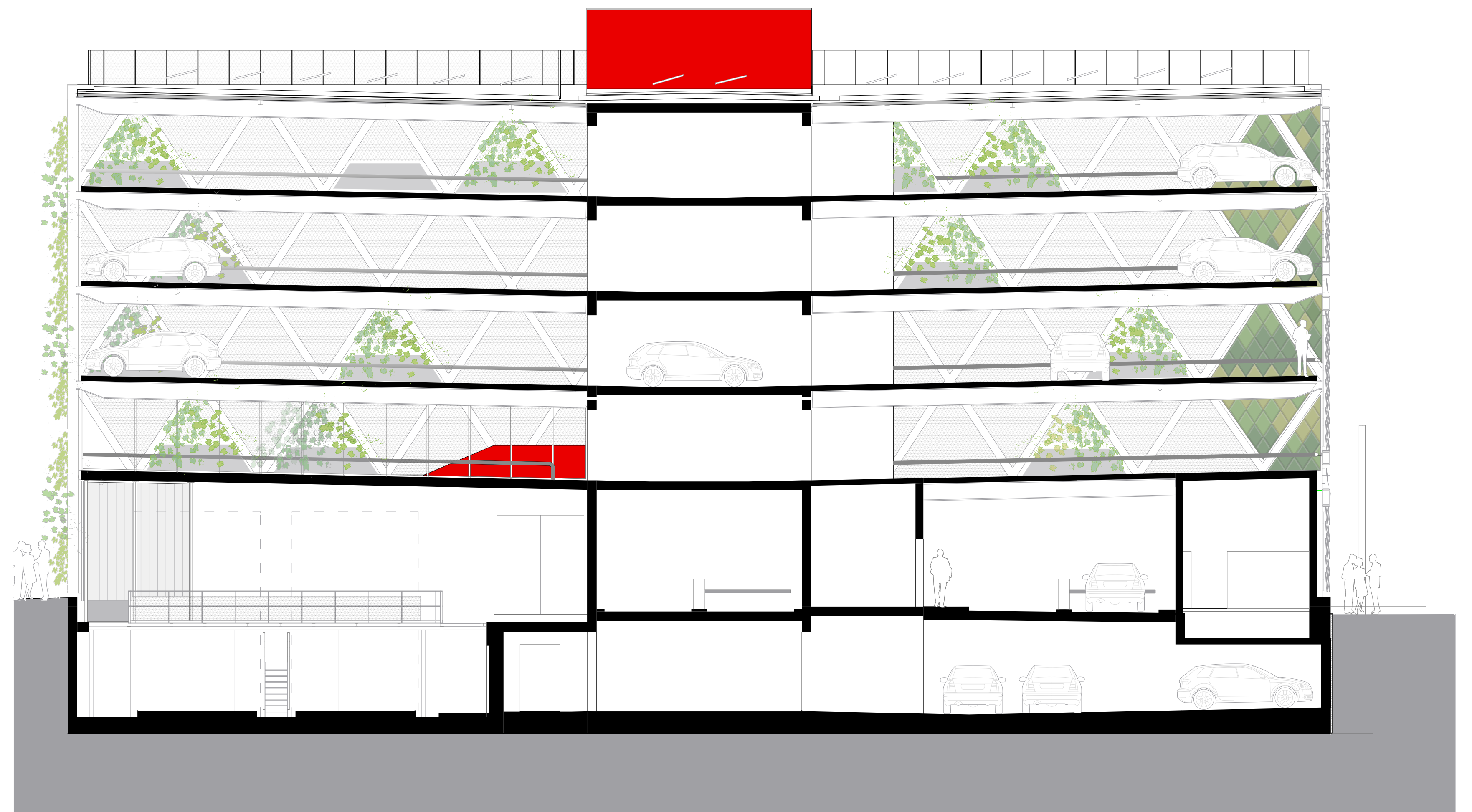
Schnitt B-B 1:100
