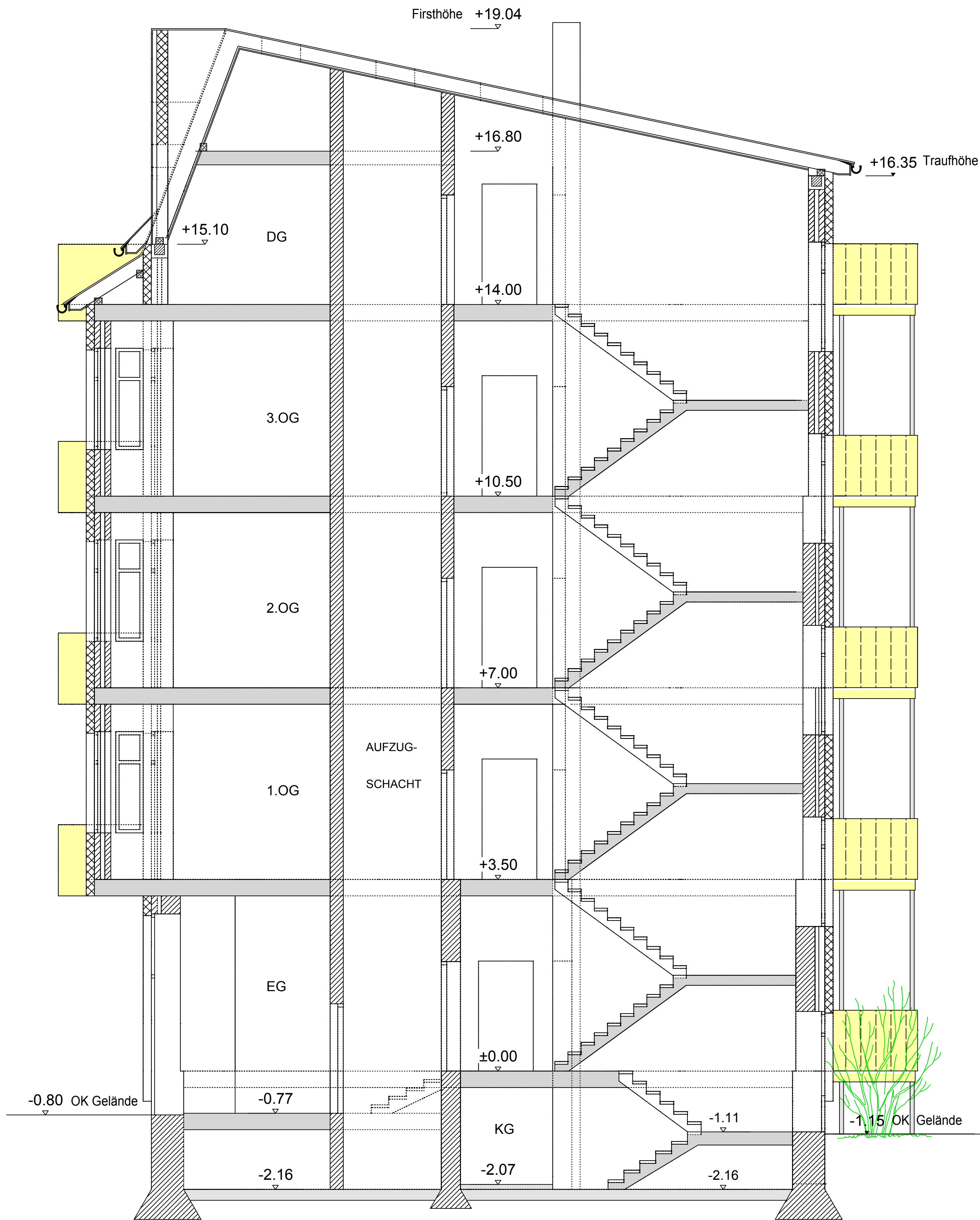
QUERSCHNITT 1: 50
