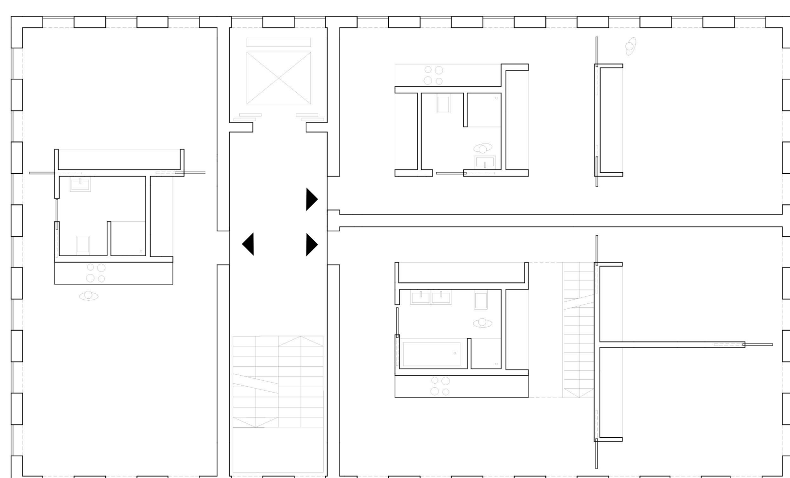
1. obergeschoss | m 1:100
