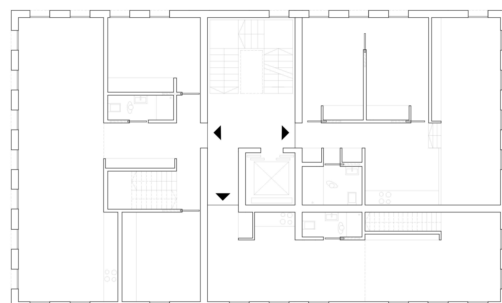
1. obergeschoss | m 1:100
