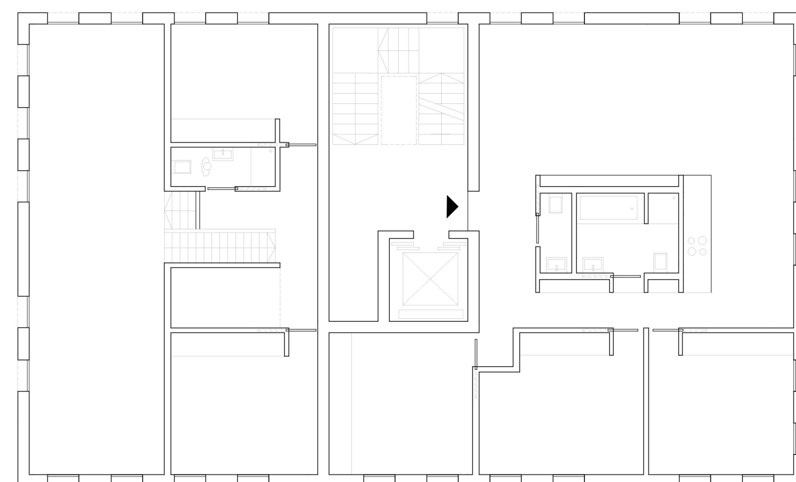
3. obergeschoss | m 1:100
