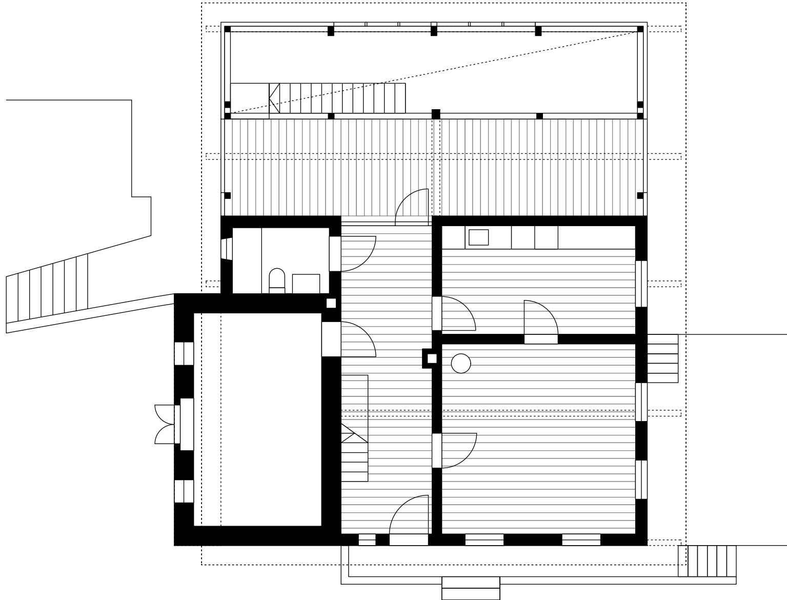
Grundriss EG
