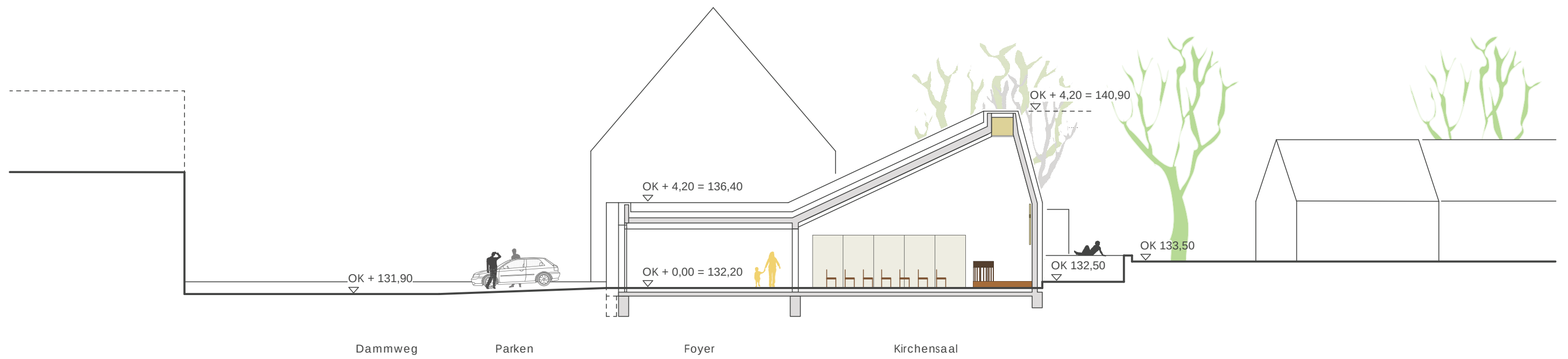
Schnitt M.1:200
