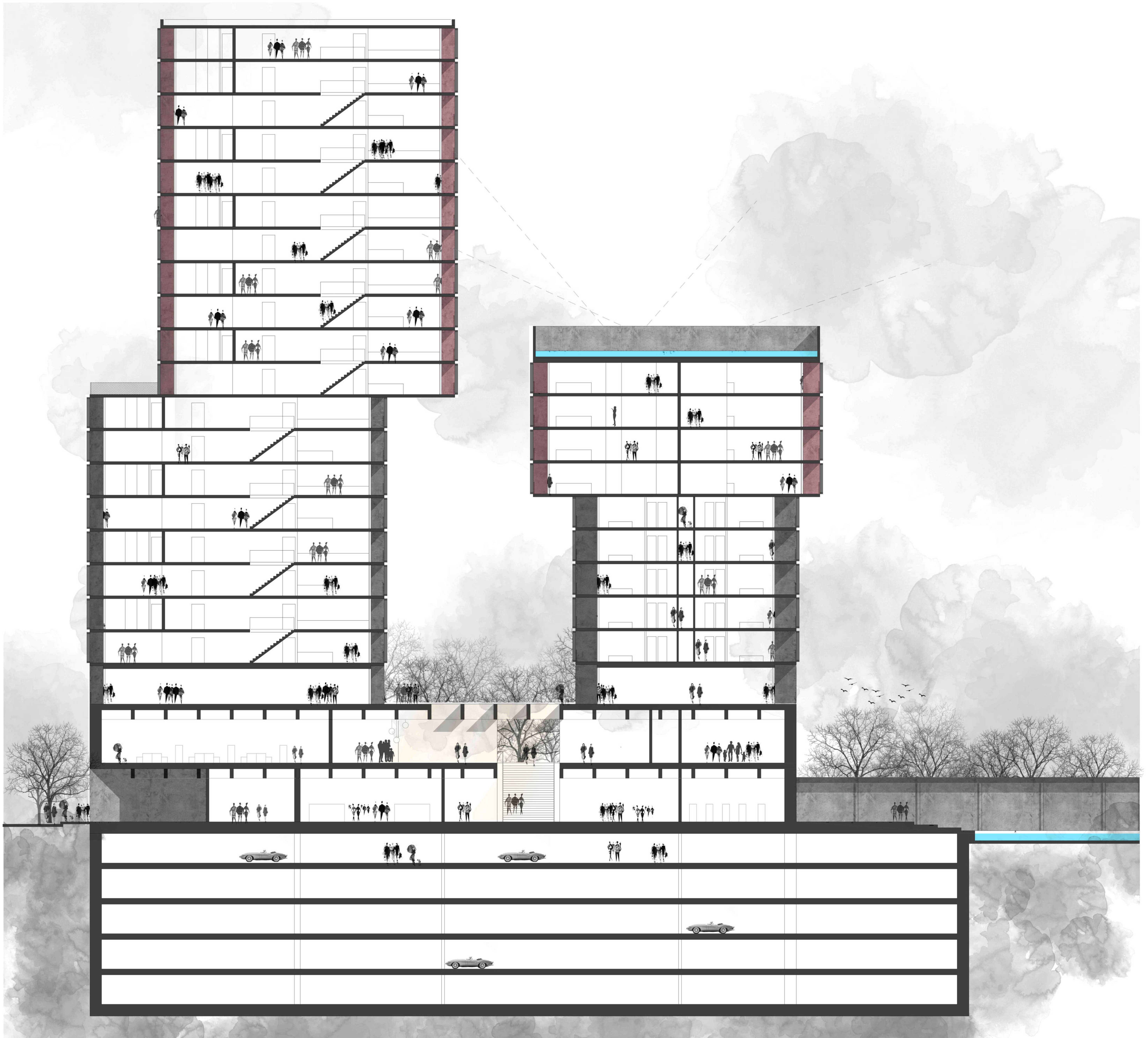
M_125 Schnitt AA
