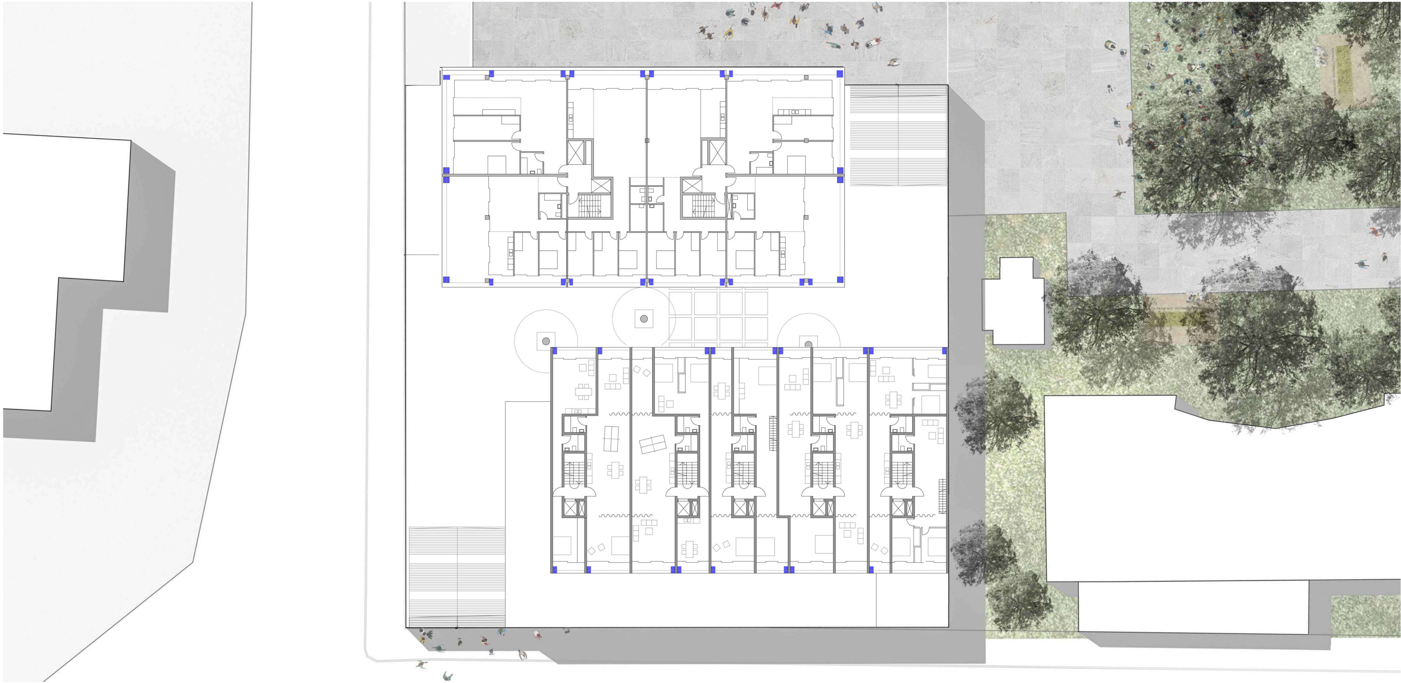
M_200 Grundriss Variante Versprung
