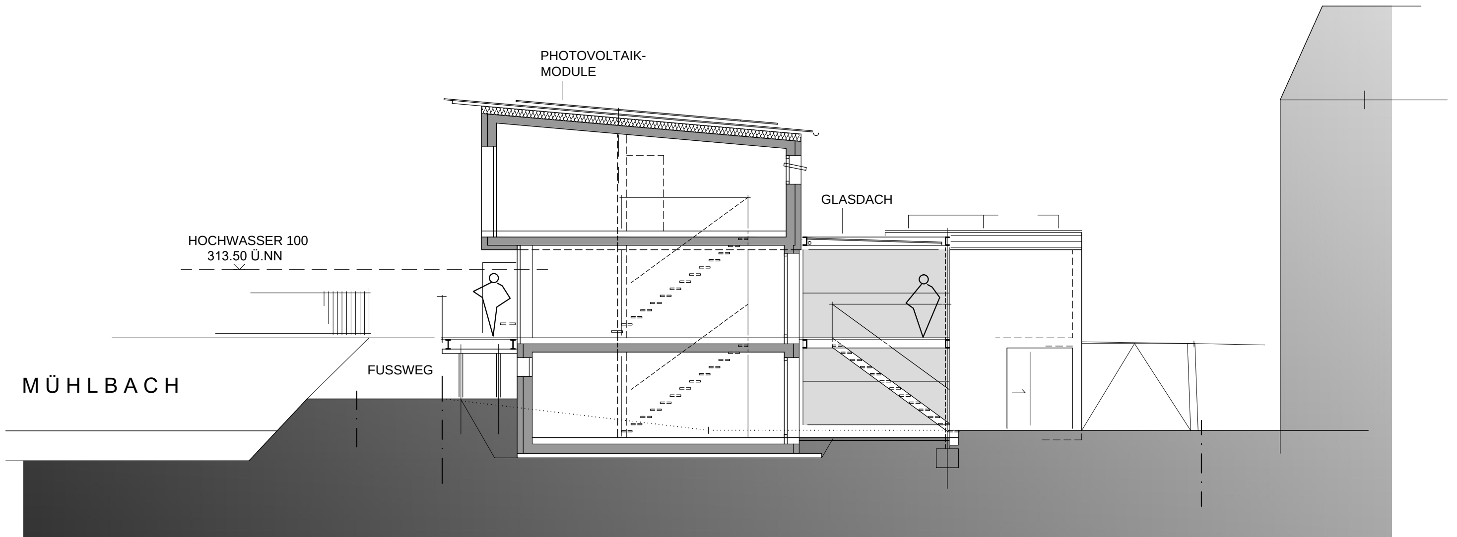
SCHNITT A-A
