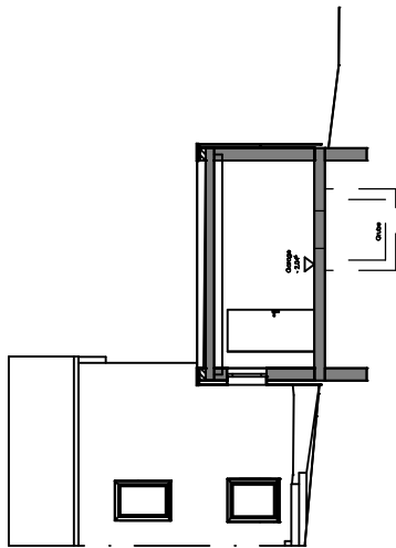
Schnitt C-C
