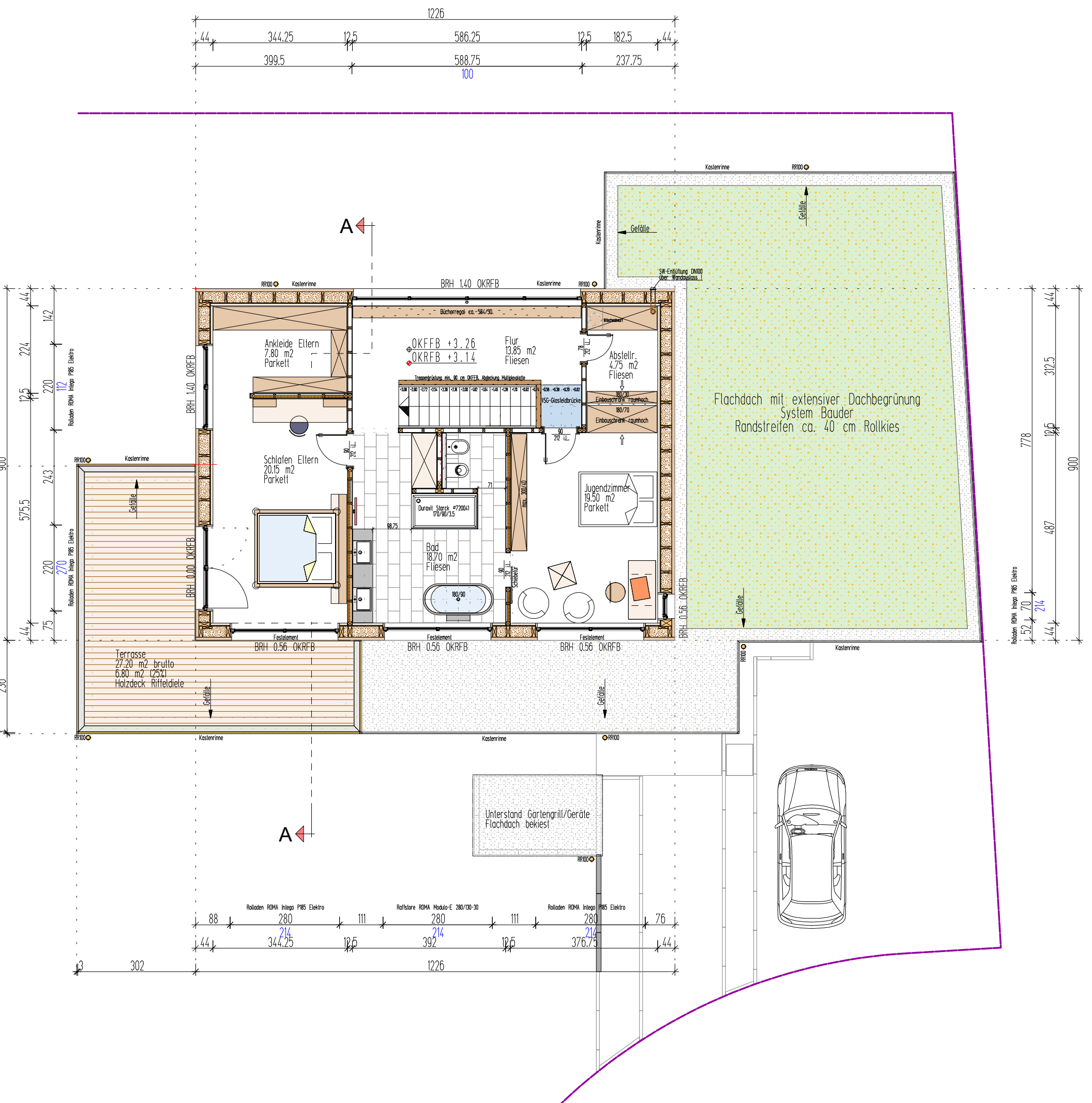
Grundriß M 1:100
