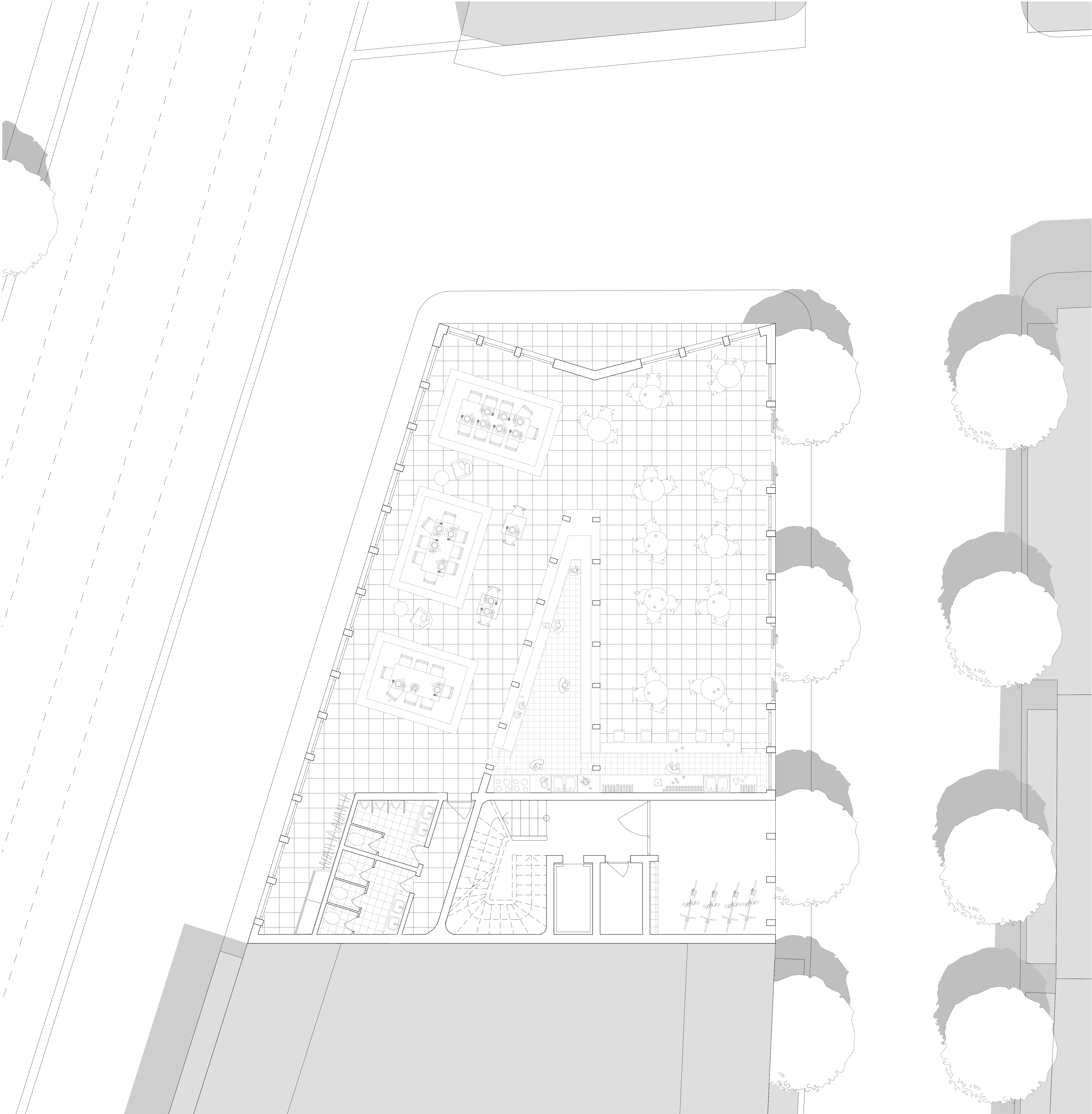
Erdgeschoss 1:50
