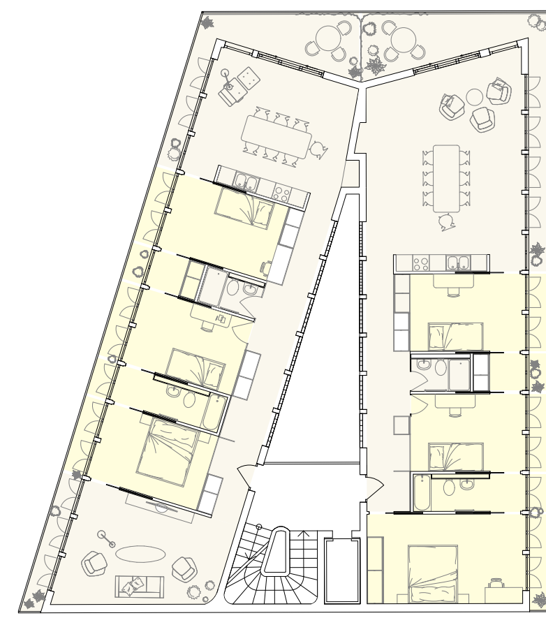
Schema Räume im Sommer
