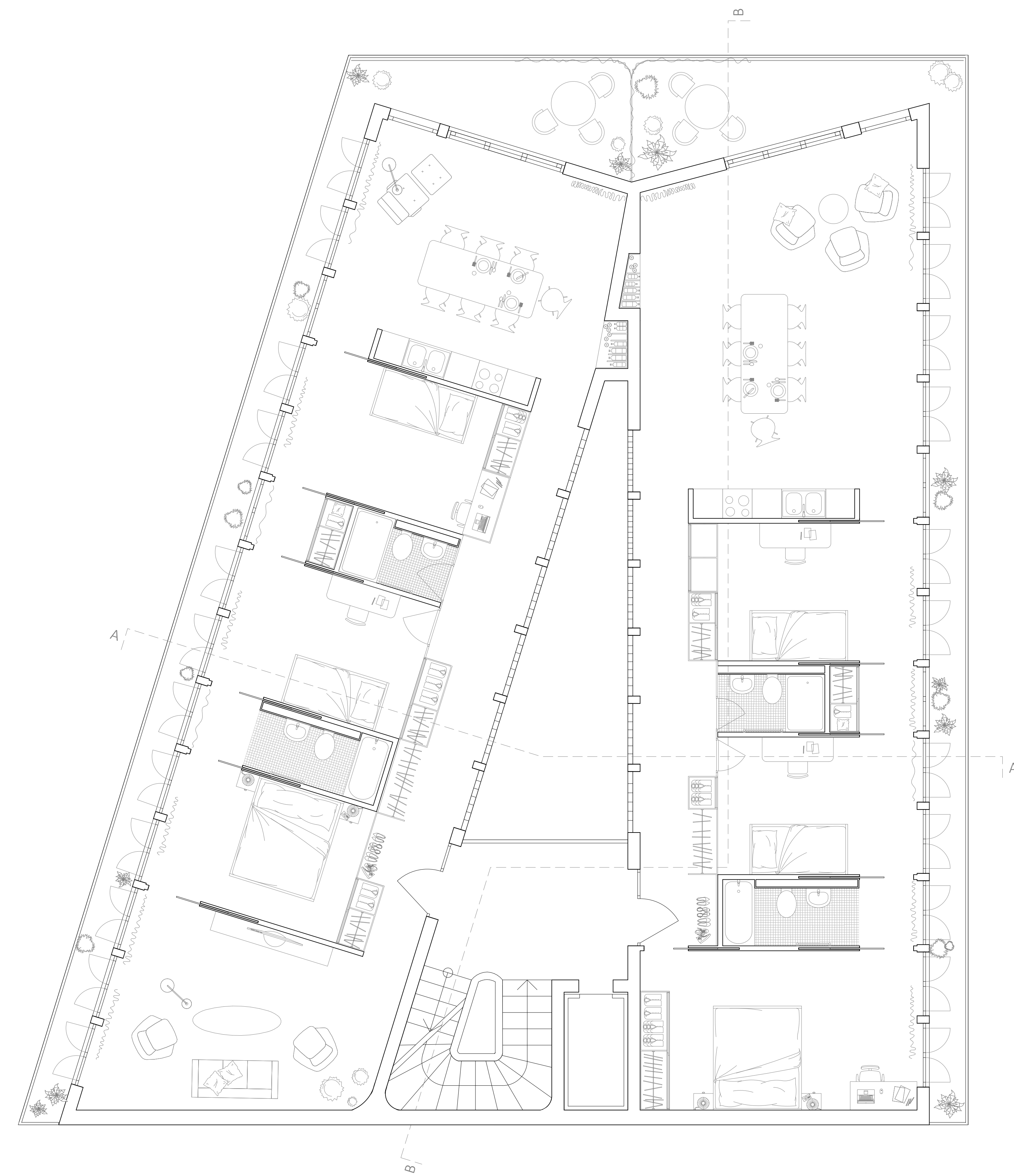
Regelgeschoss 1:50
