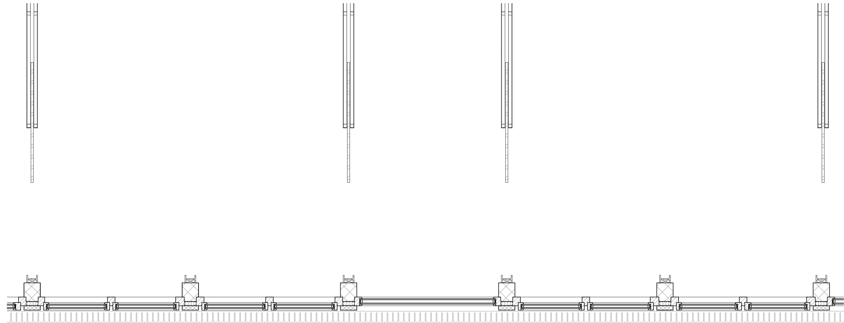
Horizontalschnitt Fassade 1:20
