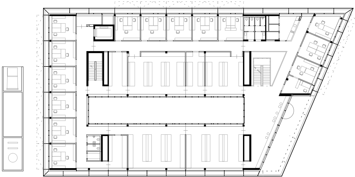
Grundriss 1.OG
