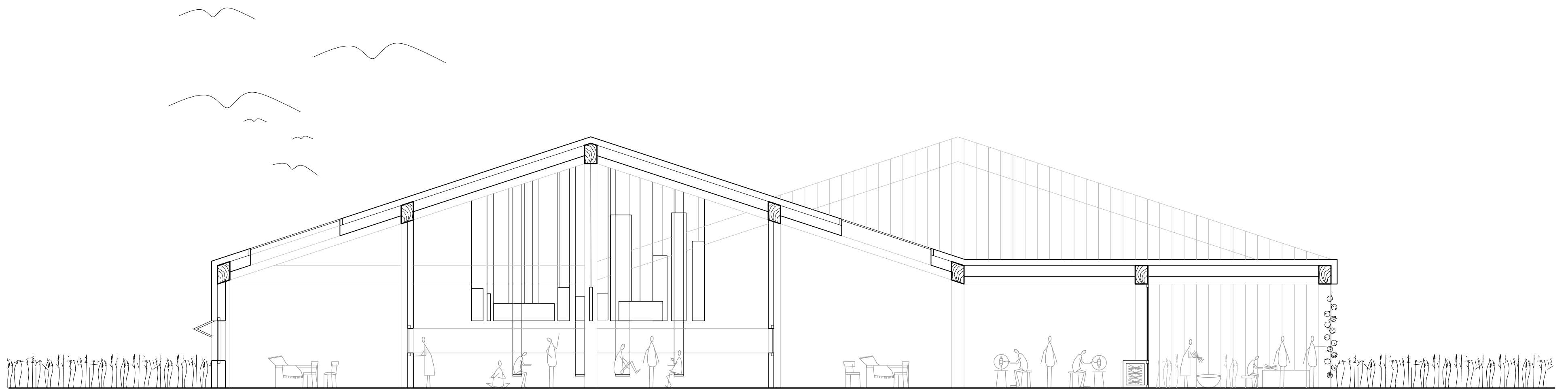
Schnitt AA, 1:100
