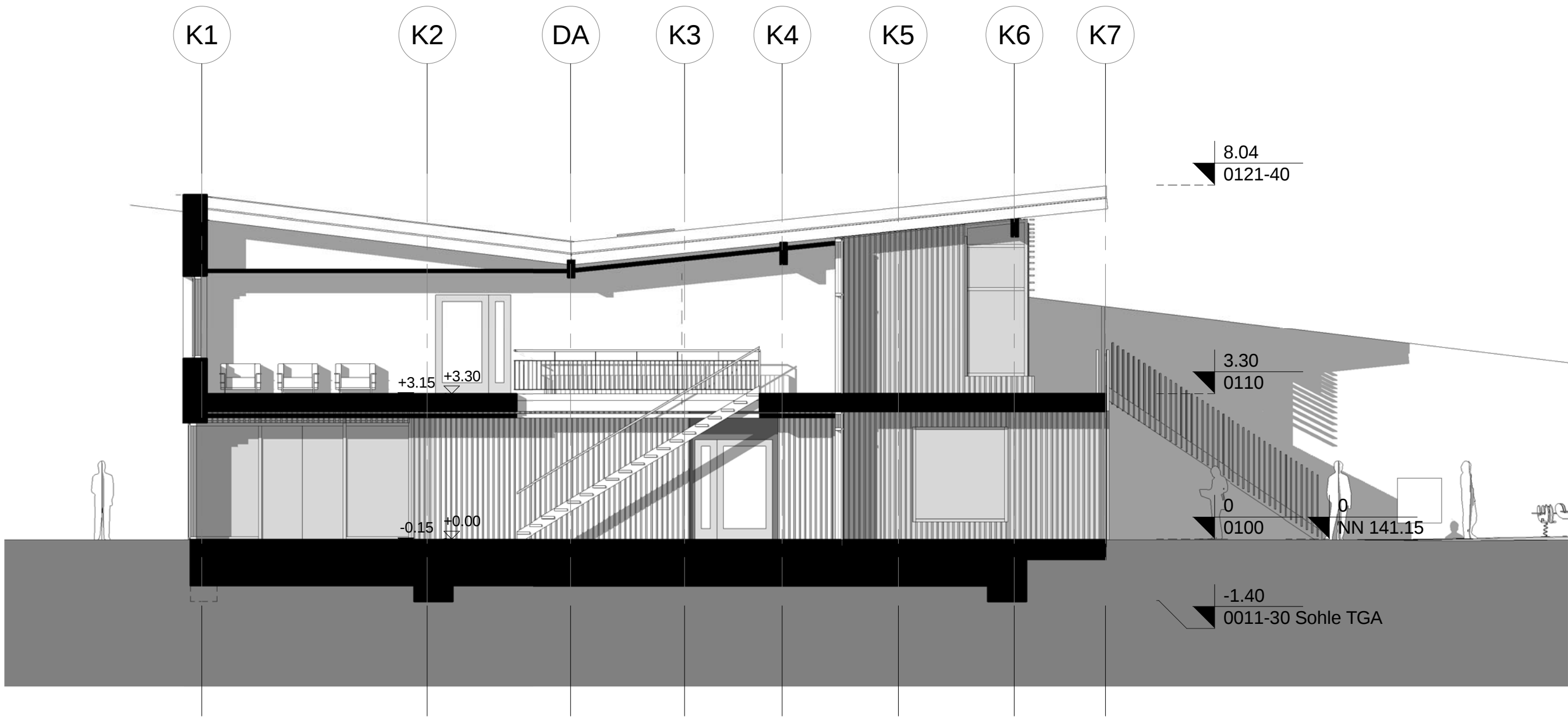
Querschnitt B-B
