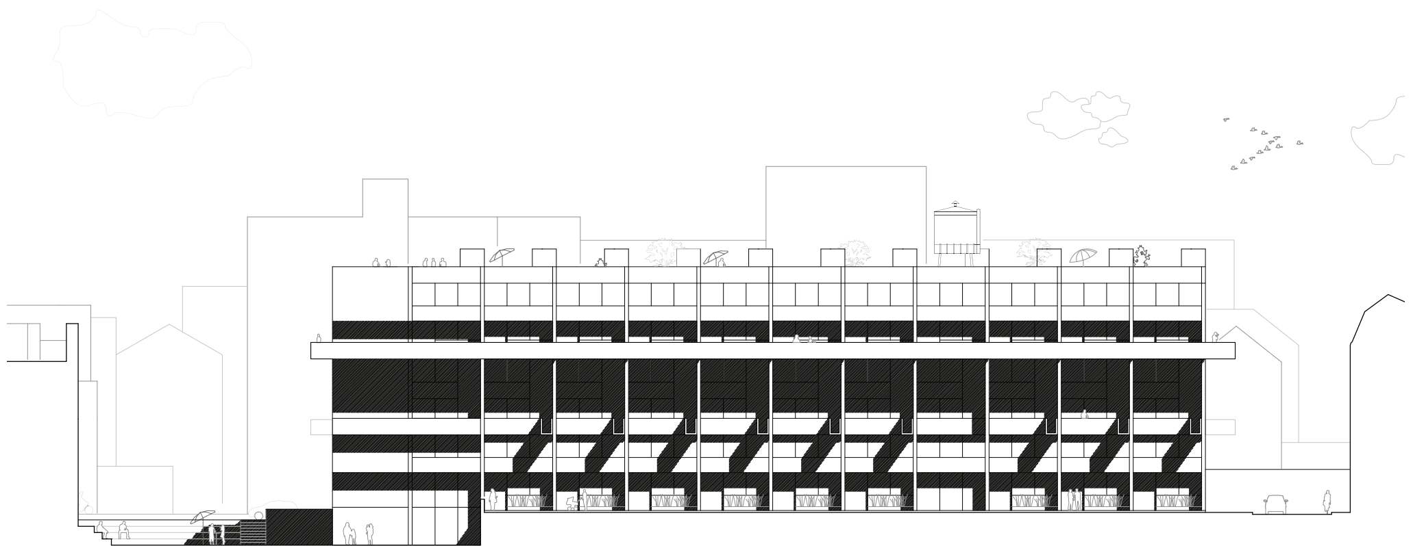
Ansicht Ost
