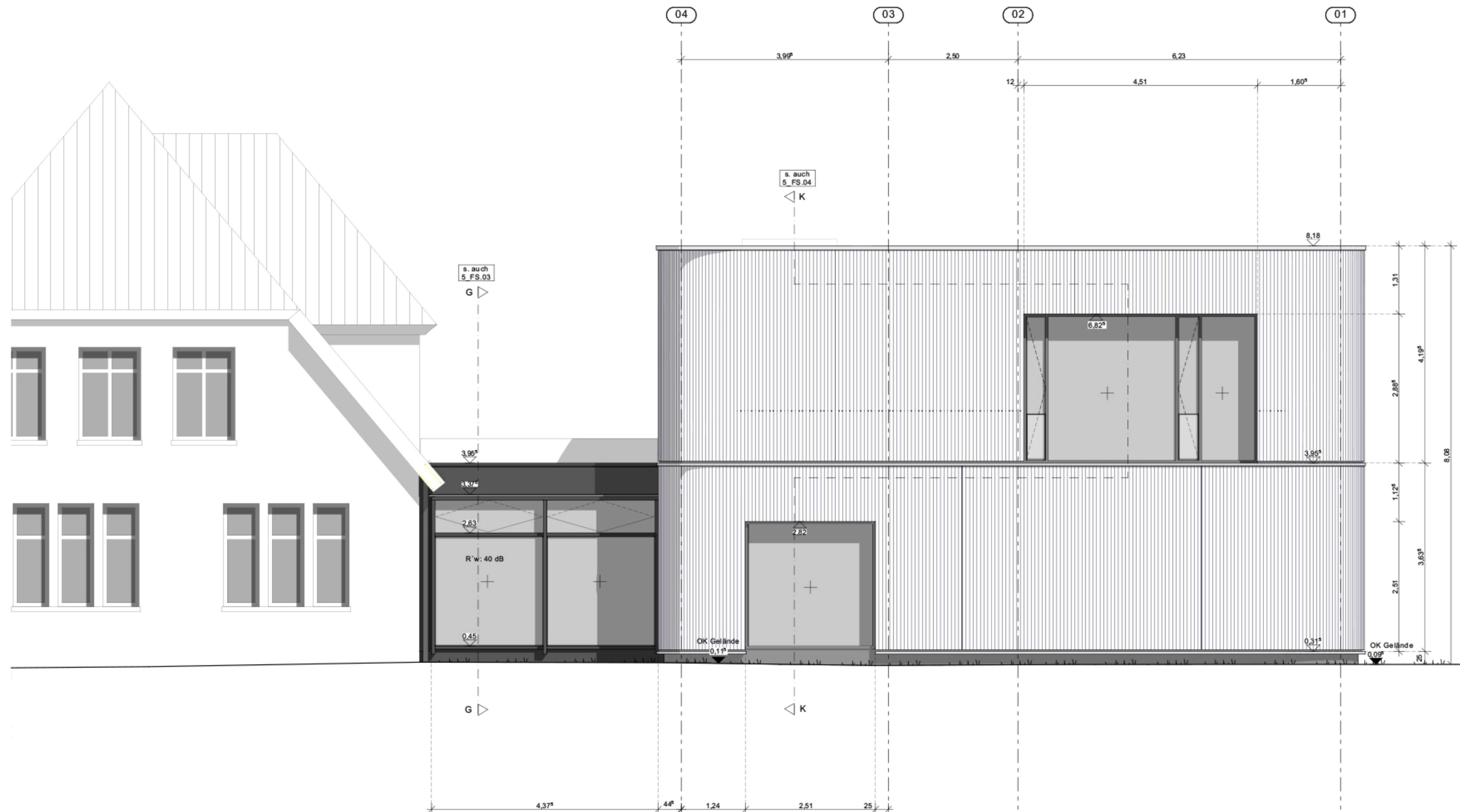
Ansicht Nord
