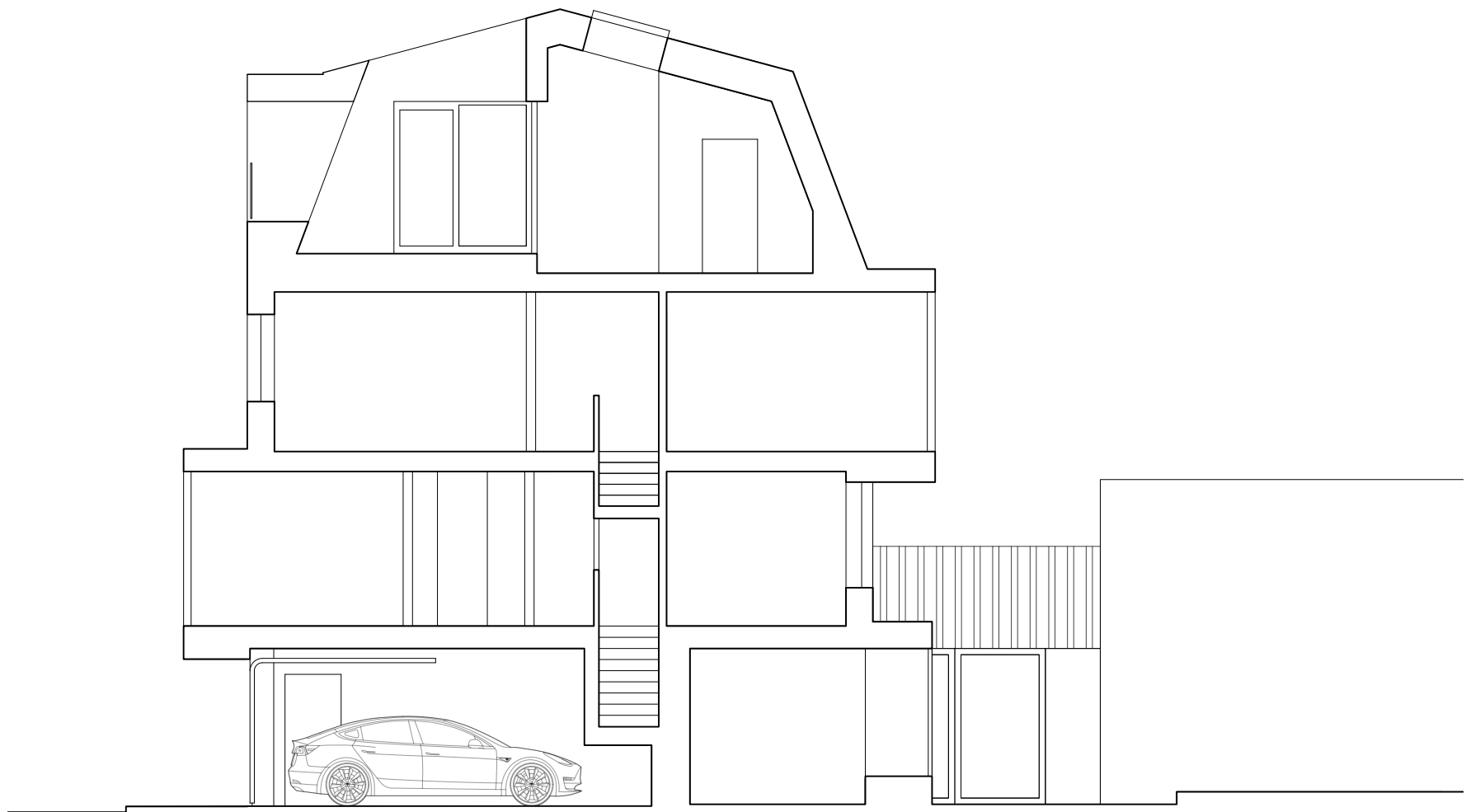
schnitt
