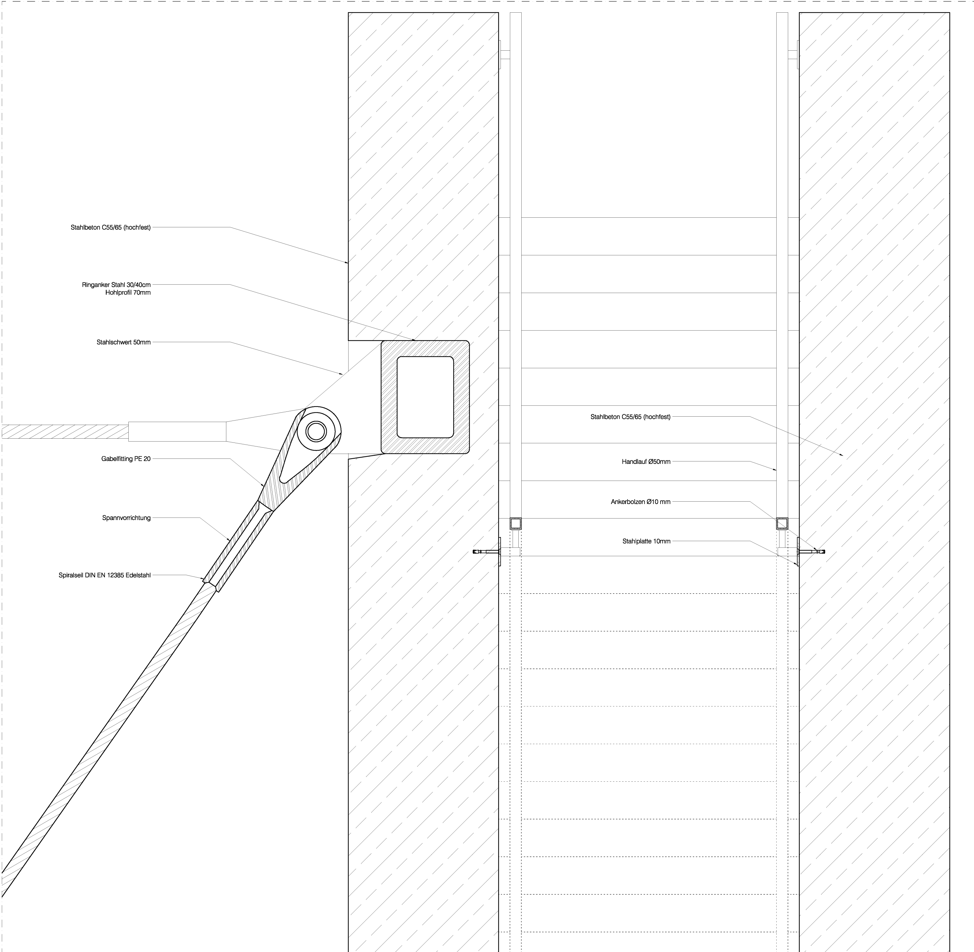
Detail Verbindung, Kugel und Wand M 1:10
