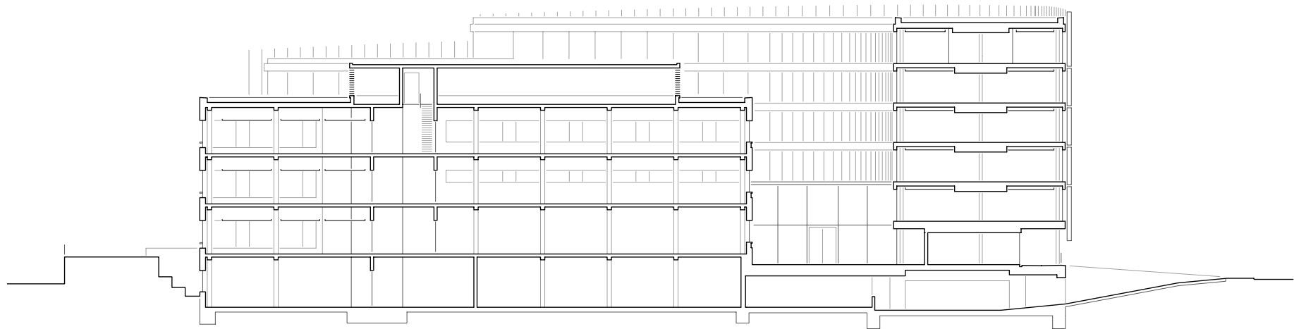
Längsschnitt
