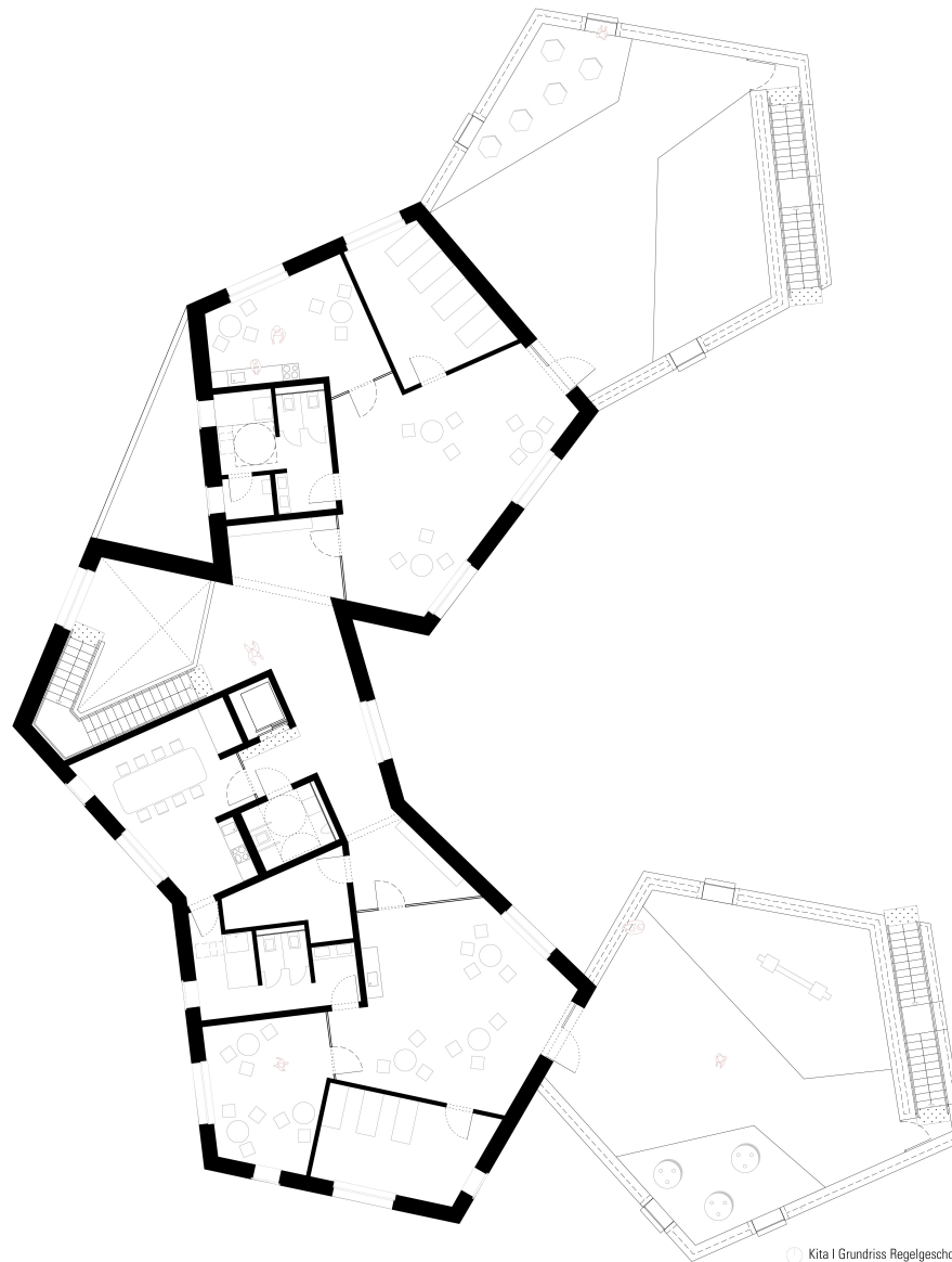
Kita I Grundriss Regelgeschoss
