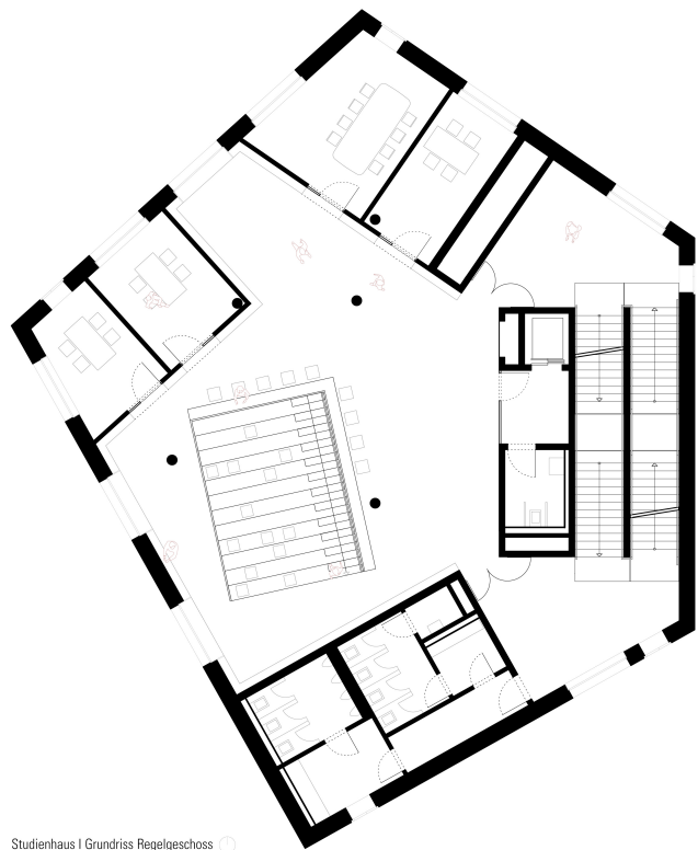
Studienhaus I Grundriss Regelgeschoss
