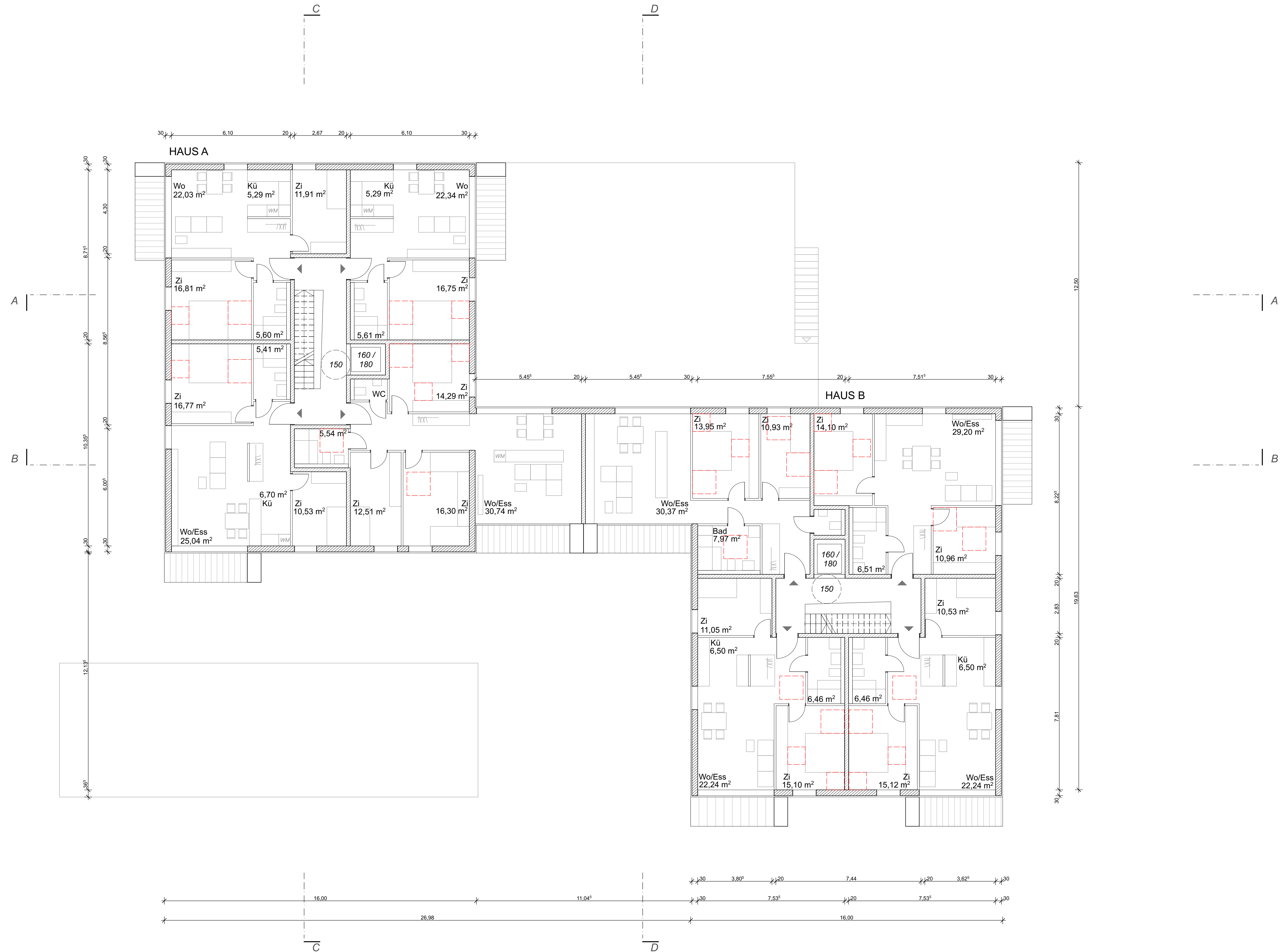
GRUNDRISS 1-2 OBERGESCHOSS 1:100
