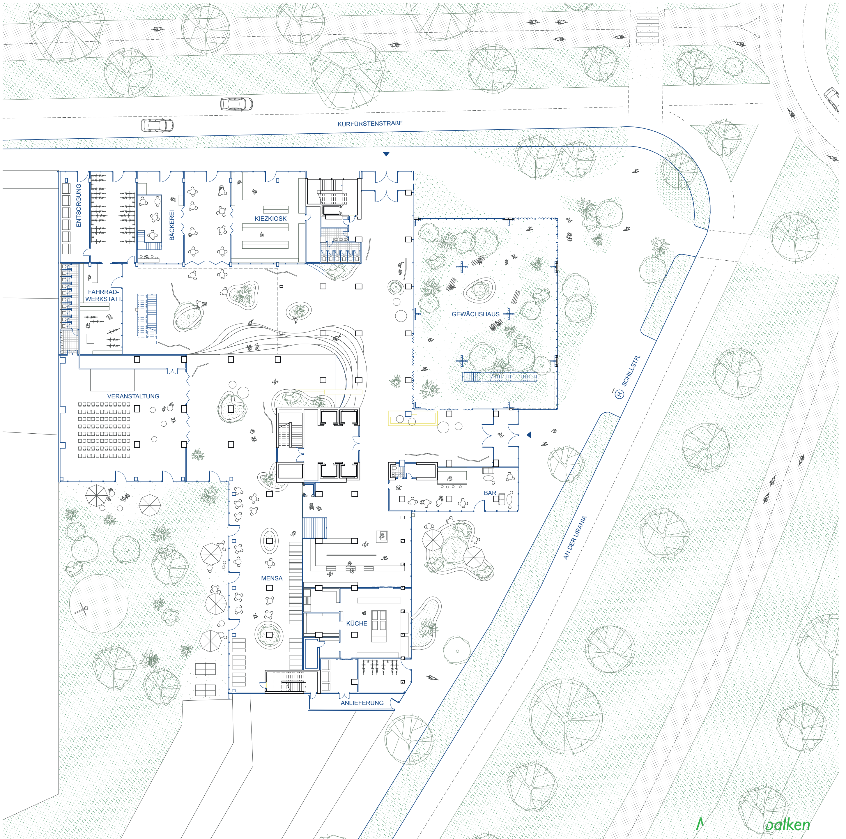
GRUNDRISS ERDGESCHOSS 1:300
