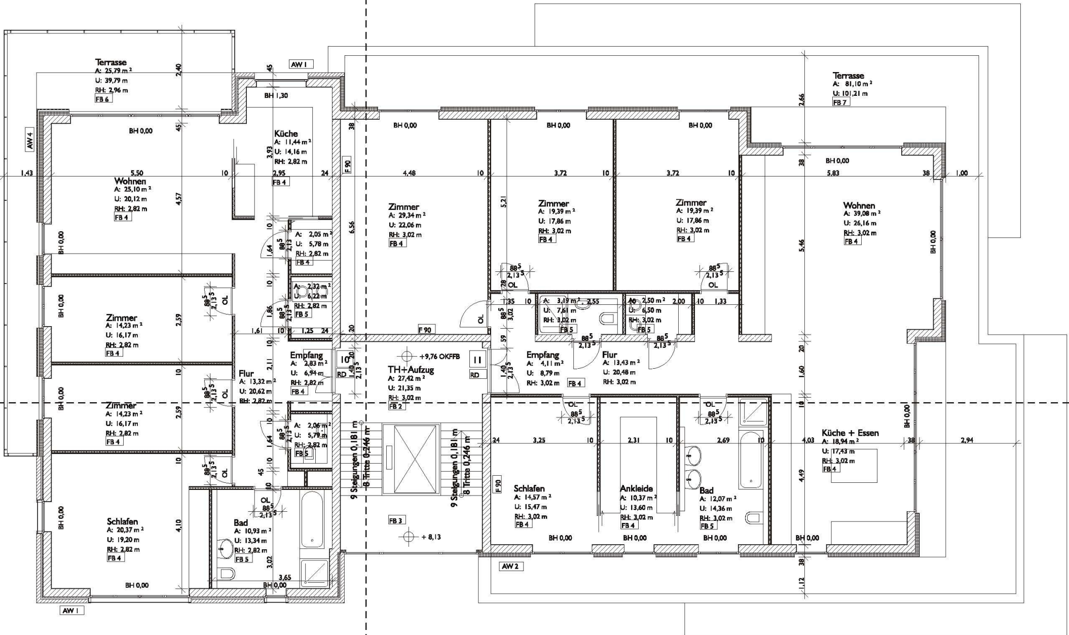
Wohnung 10 131,82 m 2
