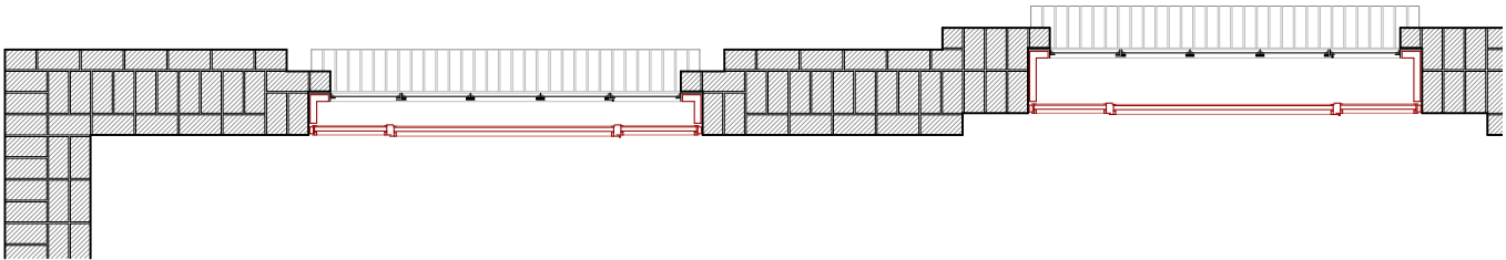
Fassade OG Vollziegel 380-510mm Ziegelflachsturz/Stahlsturz Fenster mit Einfachverglasung aus Stahlprofilen Neues Stahlfenster mit Zweifachverglasung Option Sonnenschutz in Zwischenraum Innenputz
