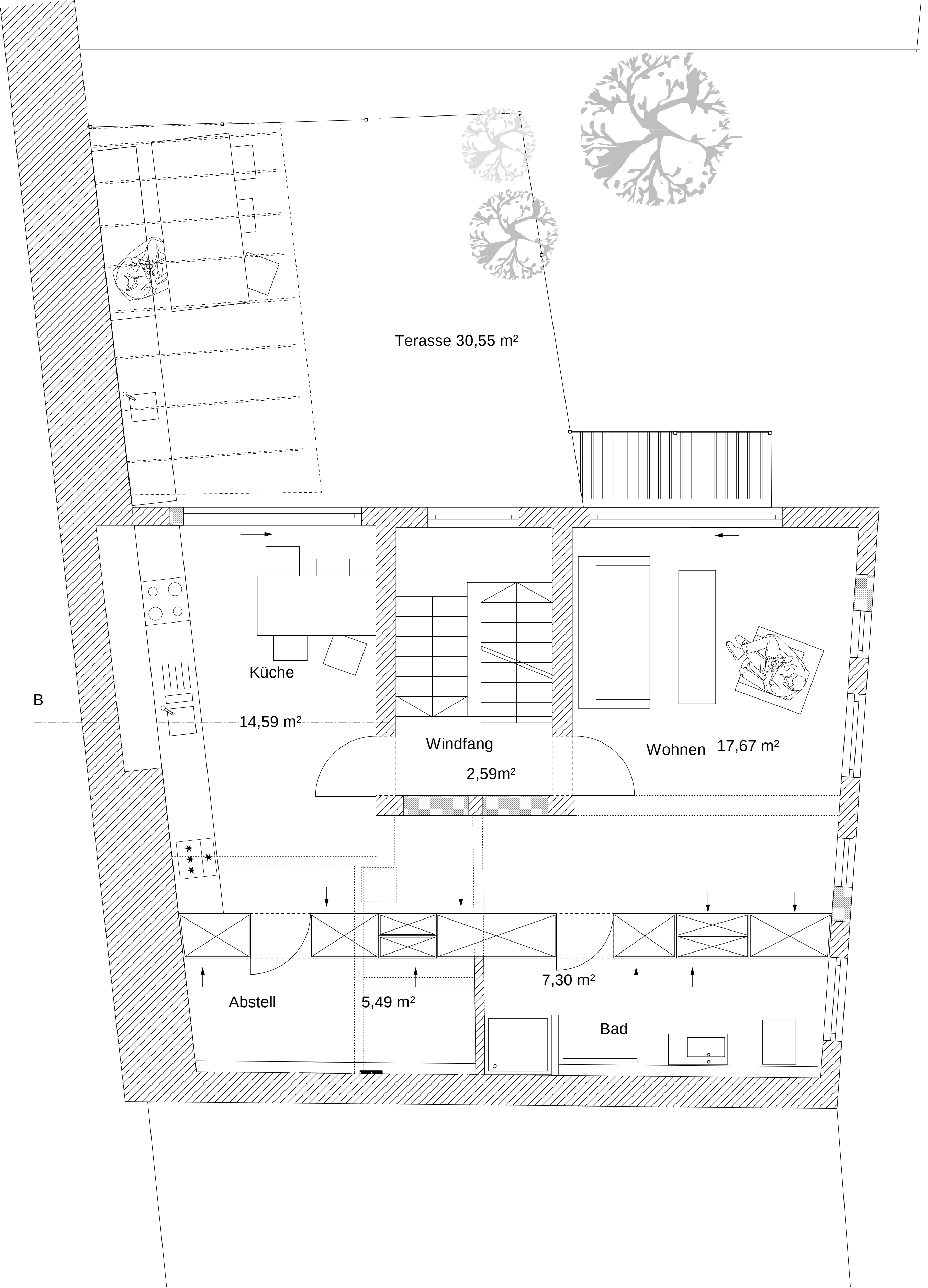
Grundriss Obergeschoss
