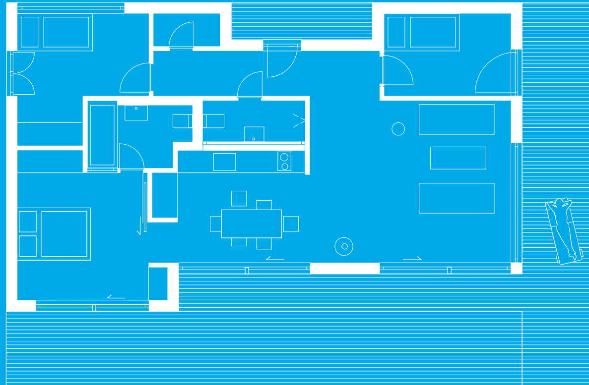
PIU 85 Grundriss | M 1:100
