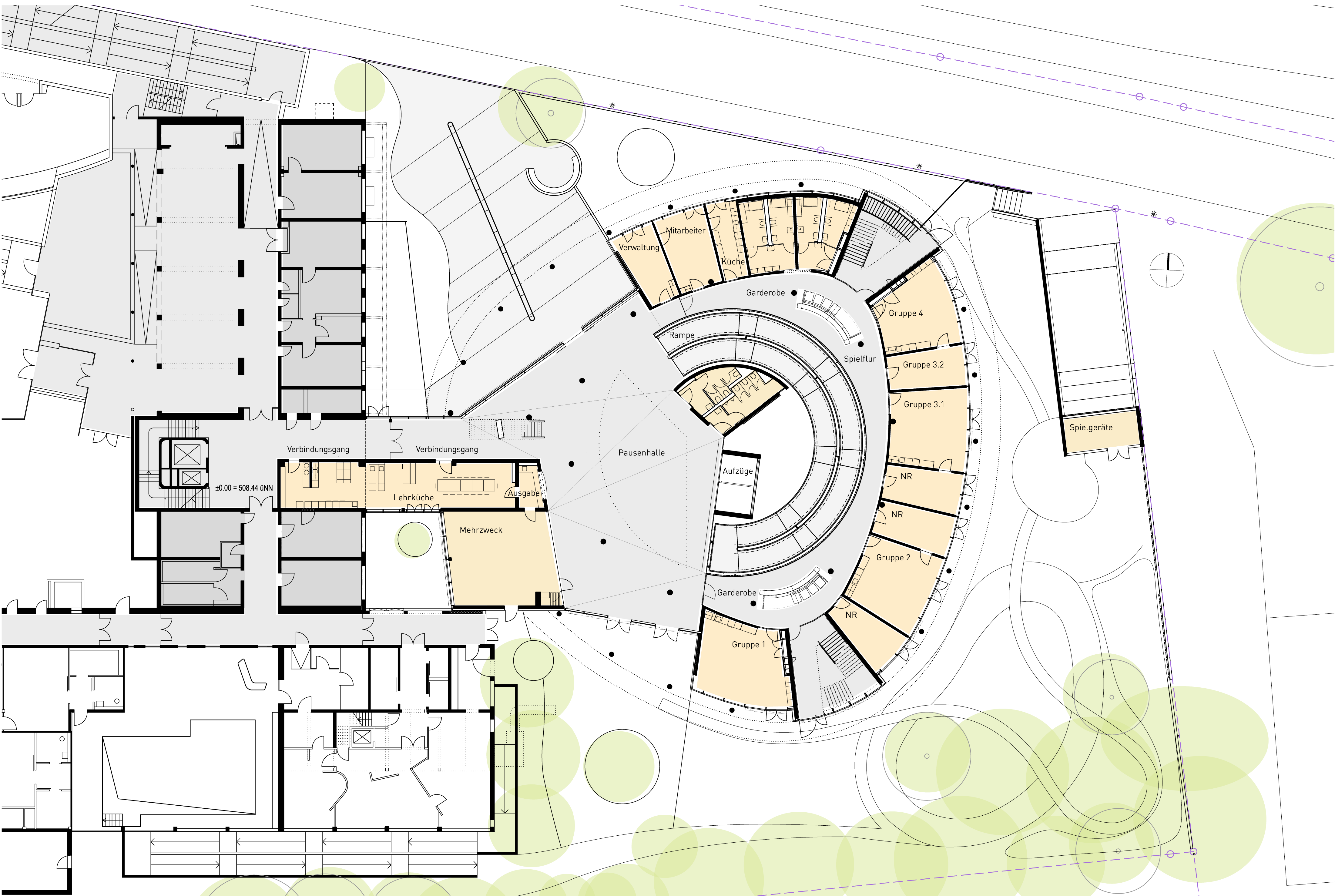
Eingangsgeschoss
