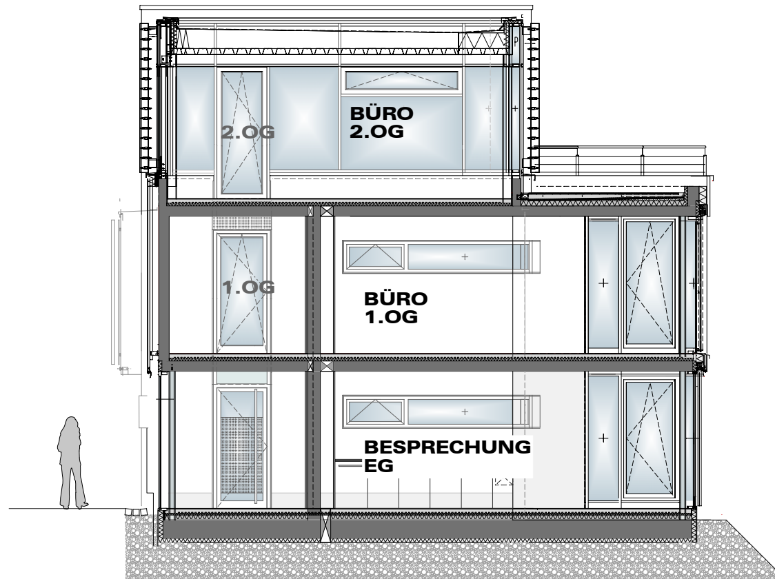
SCHNITT B-B
