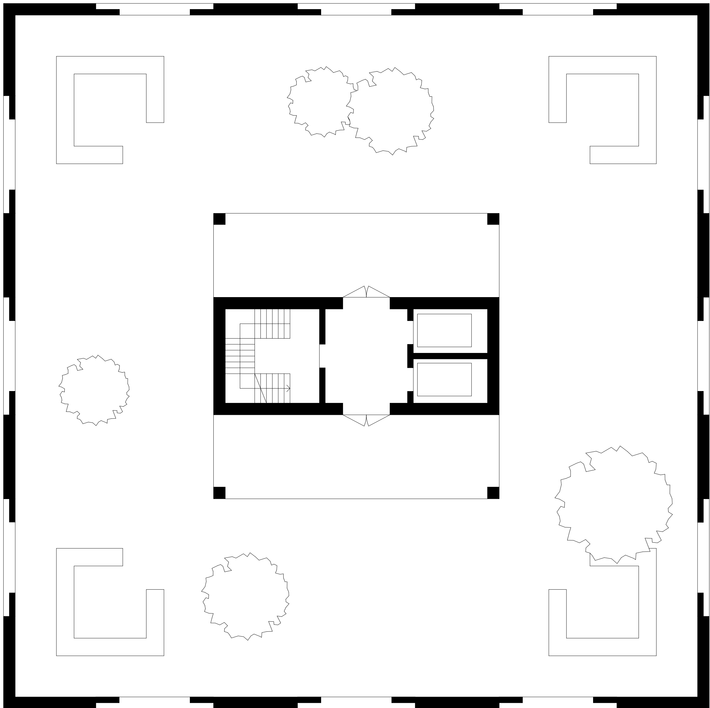
Dachgarten Hochhaus
