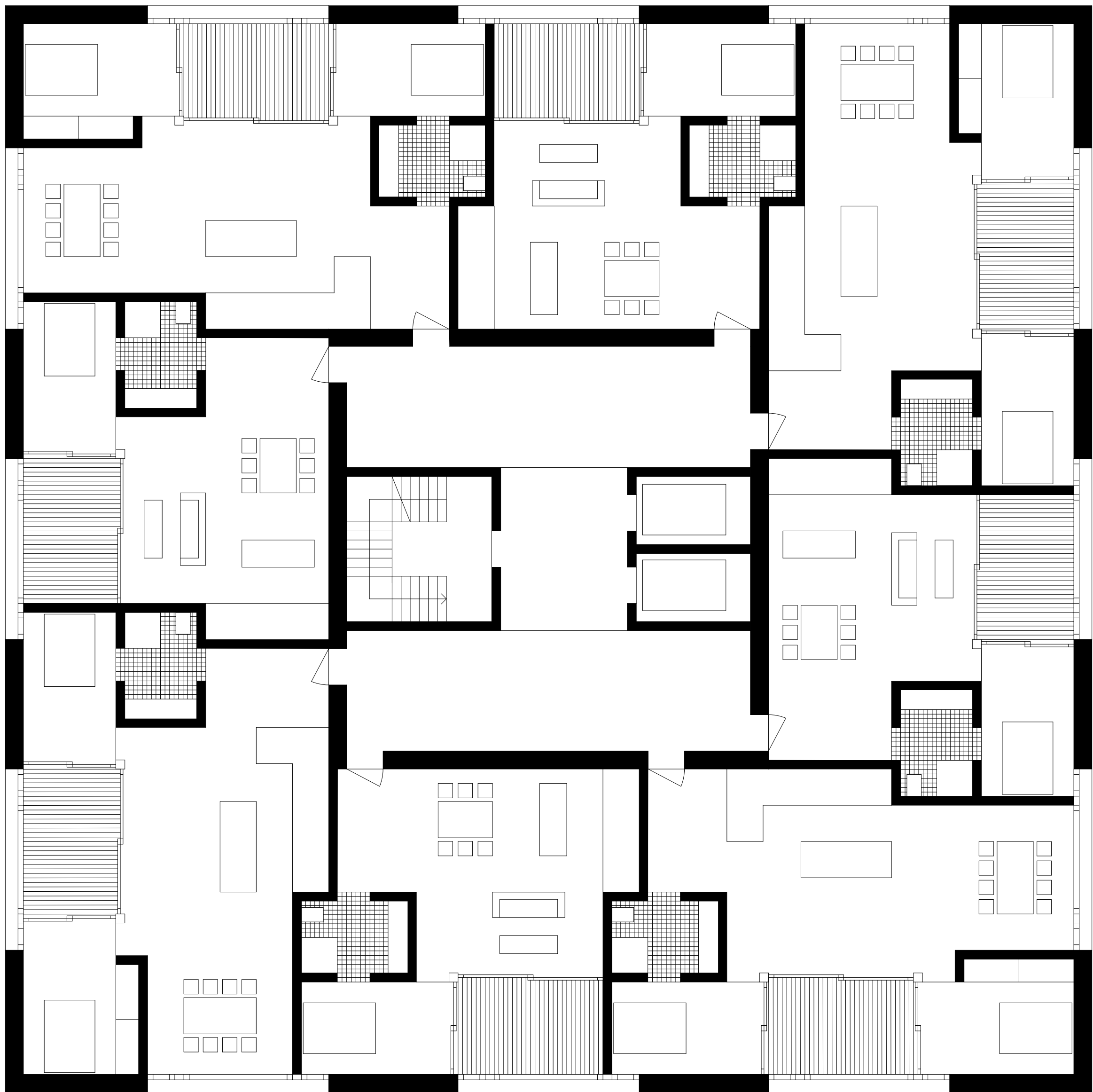
Regelgeschoss Hochhaus
