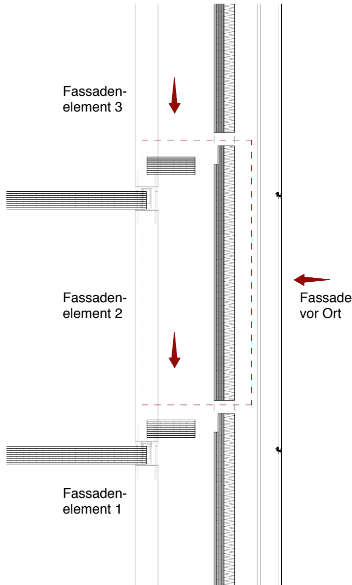
FASSADENMONTAGE
