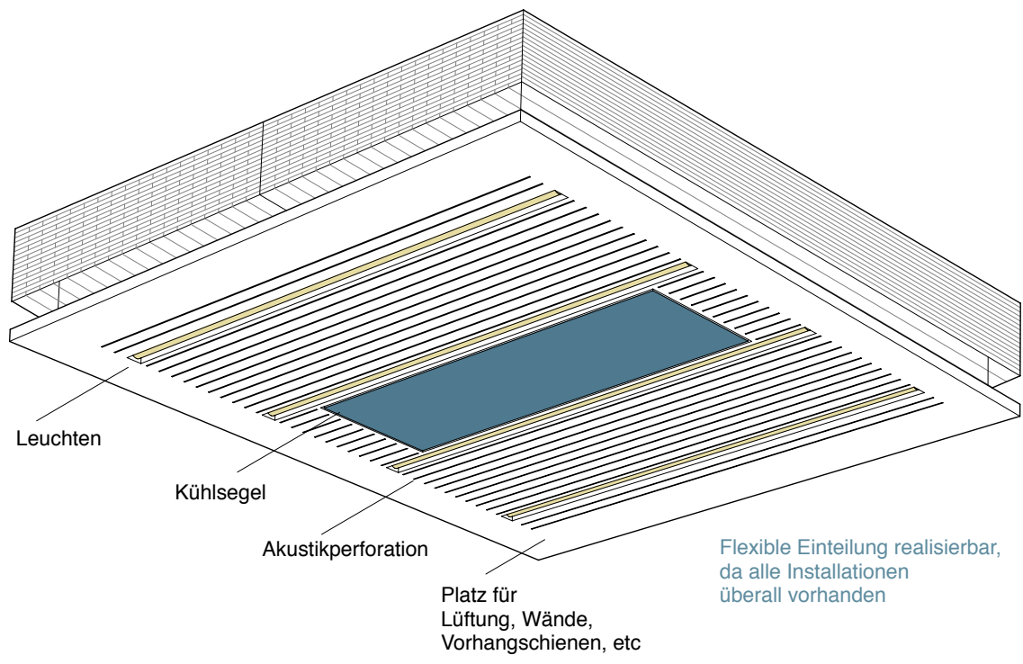
MULTIFUNKTIONALES DECKENELEMENT
