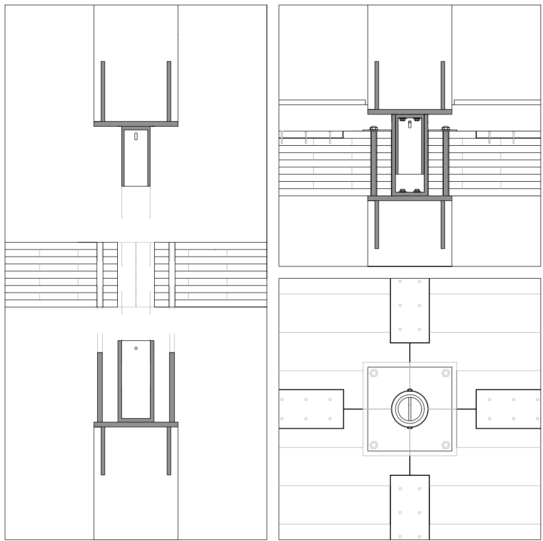
ANSCHLUSS DECKE AN STÜTZE
