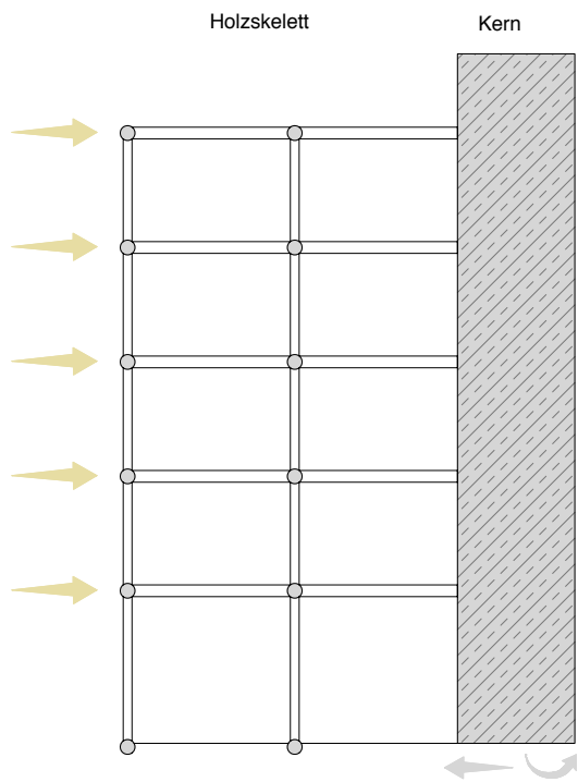
AUSSTEIFUNGSPRINZIP
