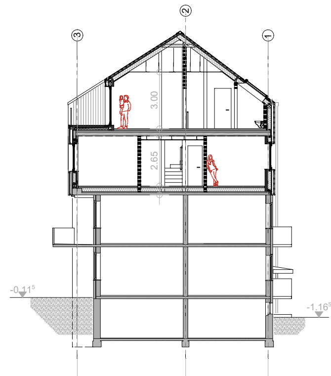
Schnitt 1:200
